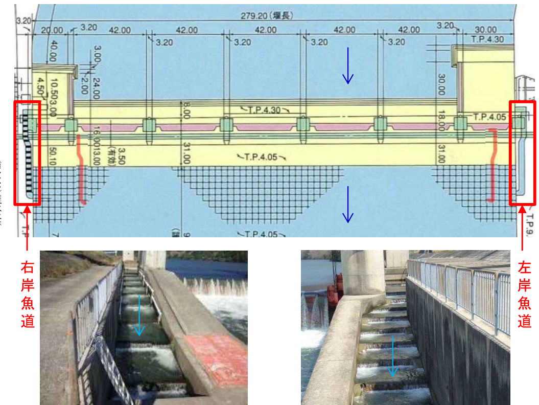
○魚道等設備の配置
