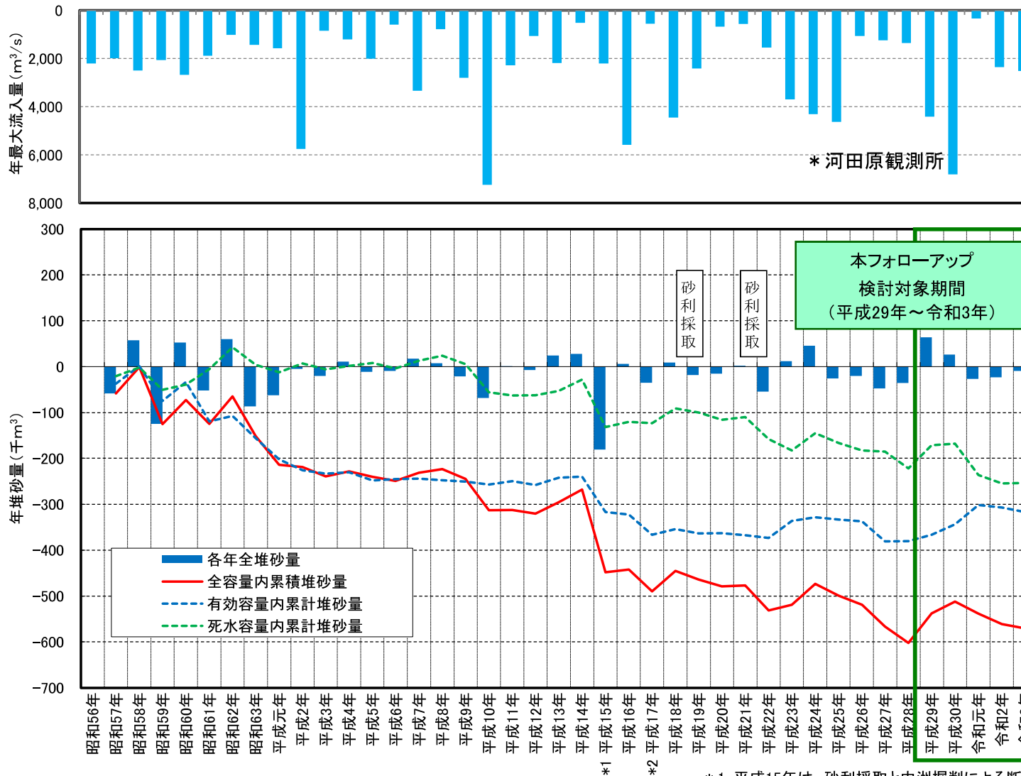
【堆砂経年変化と年最大流入量（S56～R3）】
