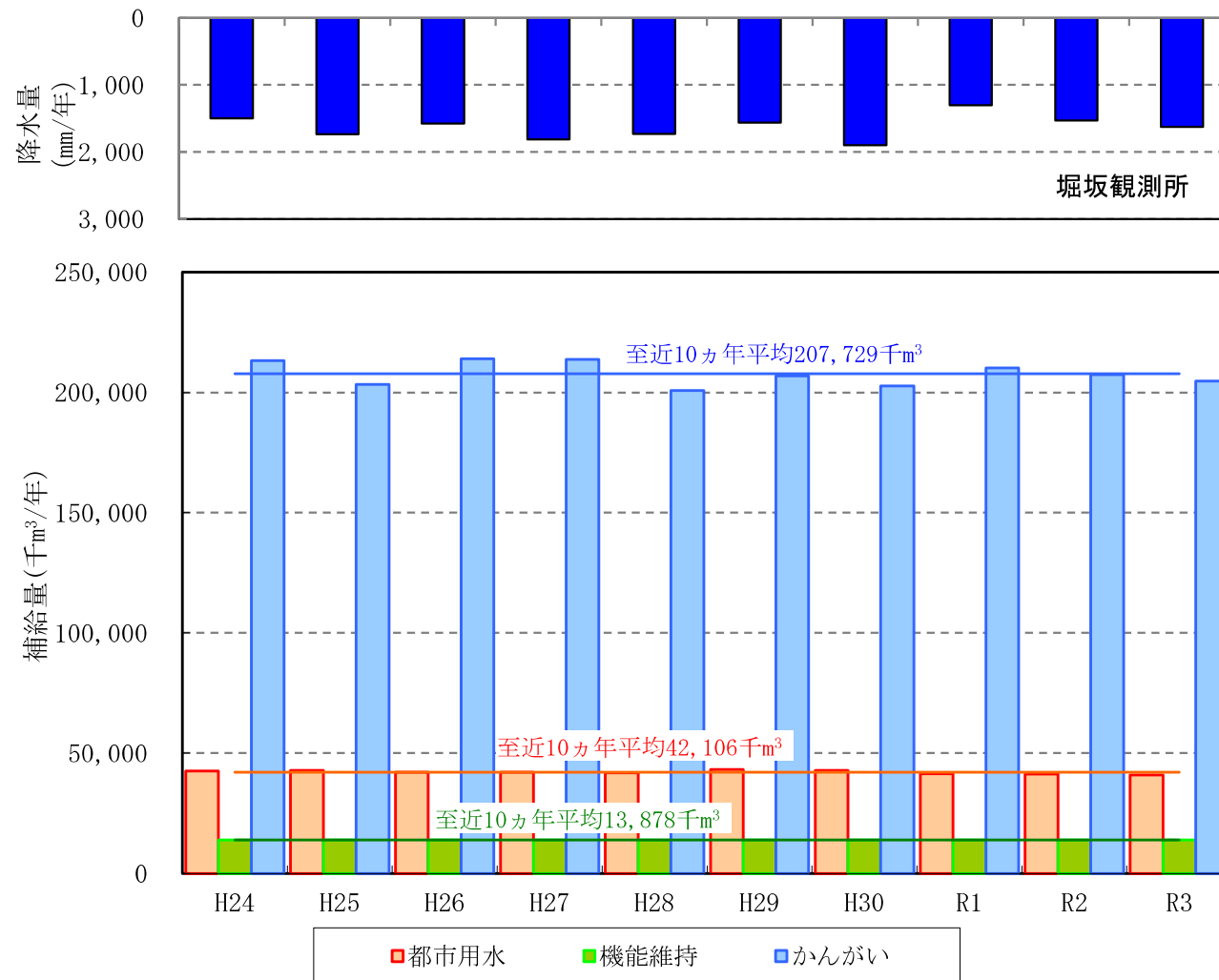
【坂根堰水源での利水補給実績】
