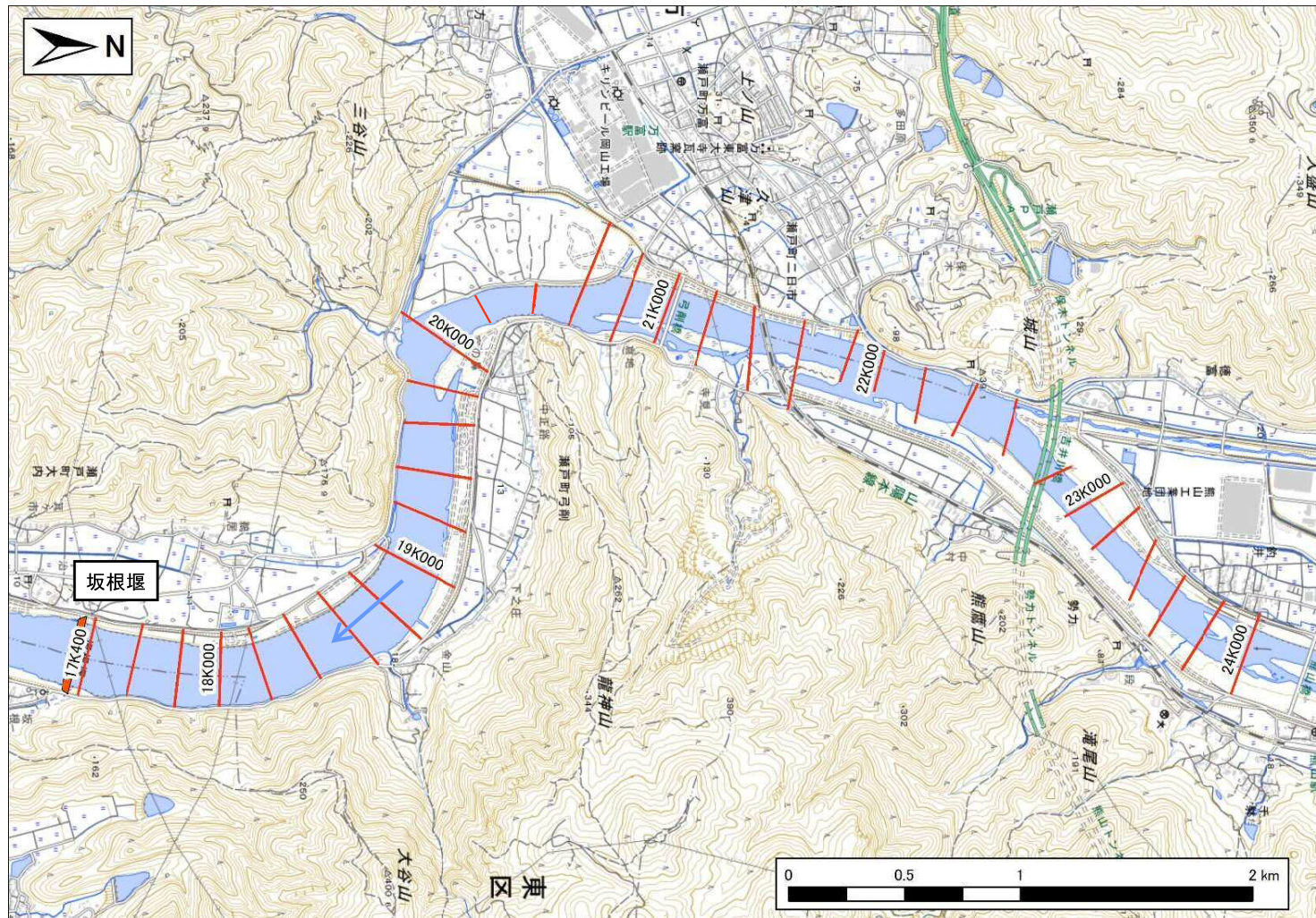
【堰周辺測量範囲位置図】
