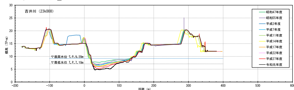
【横断図(19.8k、23k)】
