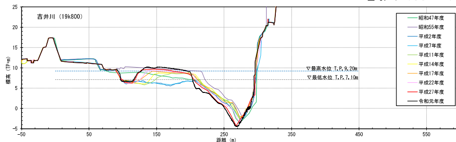
【横断図(19.8k、23k)】
