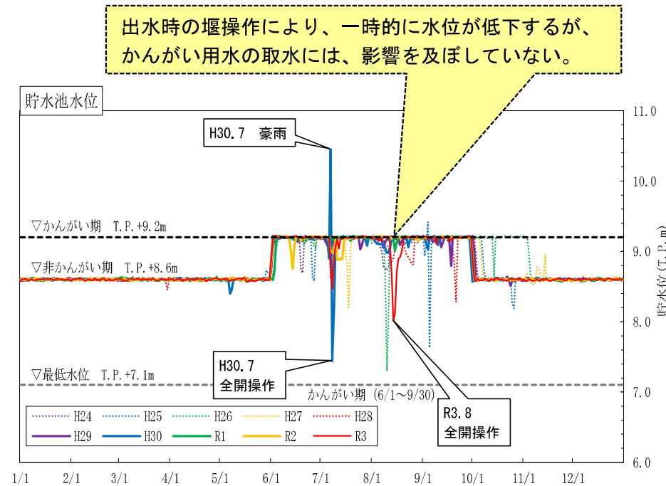
○H24～R3年（至近20年）の貯水位の変化
