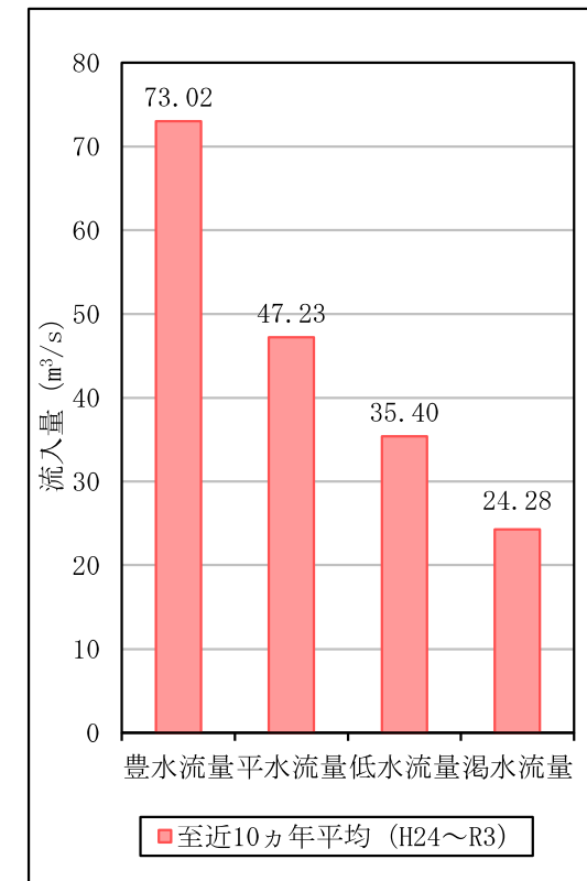
【坂根堰流入量(流況)】
