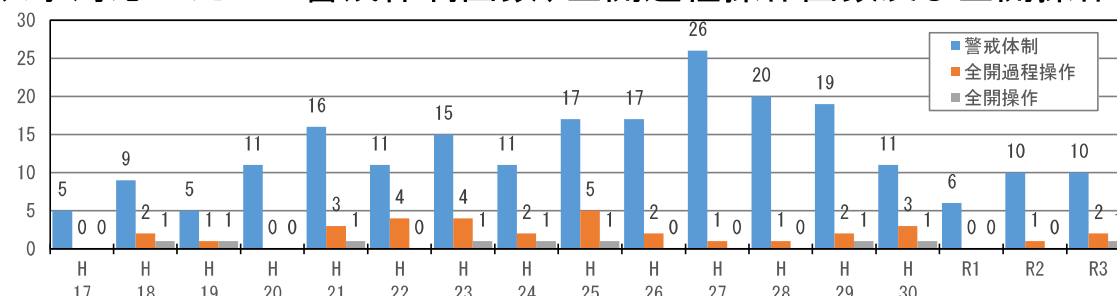
【洪水対応のための警戒体制回数、全開過程操作回数及び全開操作回数】
