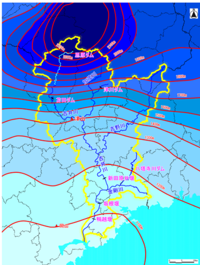
図 2.2.1 吉井川流域における年間の平均降水量分布 (昭和56年～平成22年)
