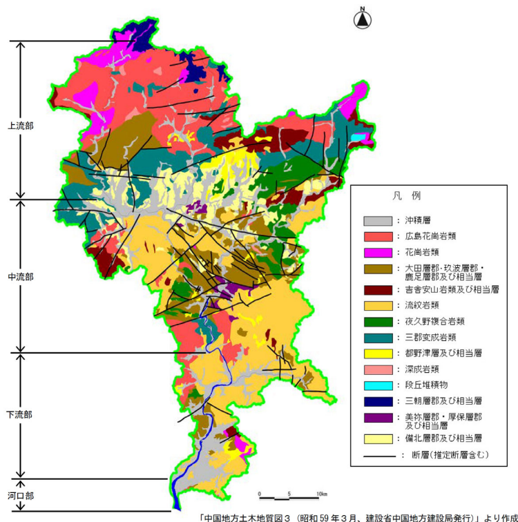
図 2.3.2 吉井川流域の地質概要図
