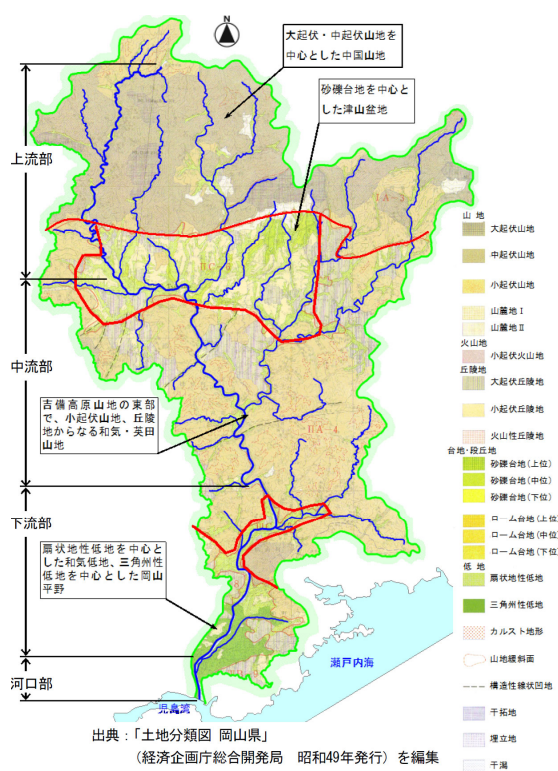
図 2.3.1 吉井川流域の地形分類図
