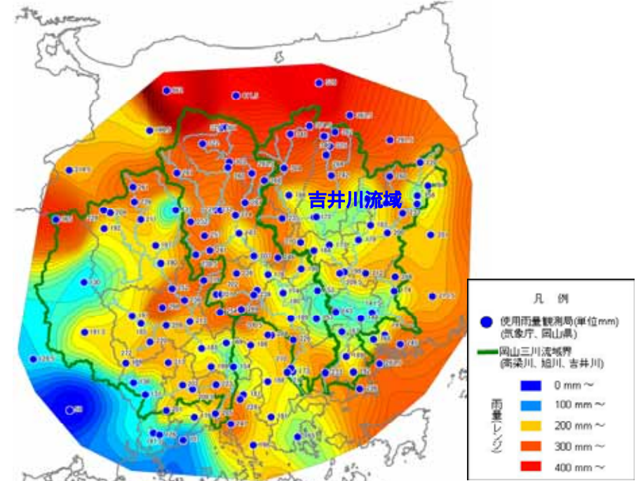
岡山県内の等雨量線図(2日雨量) [9月2日9時～4日9時]
