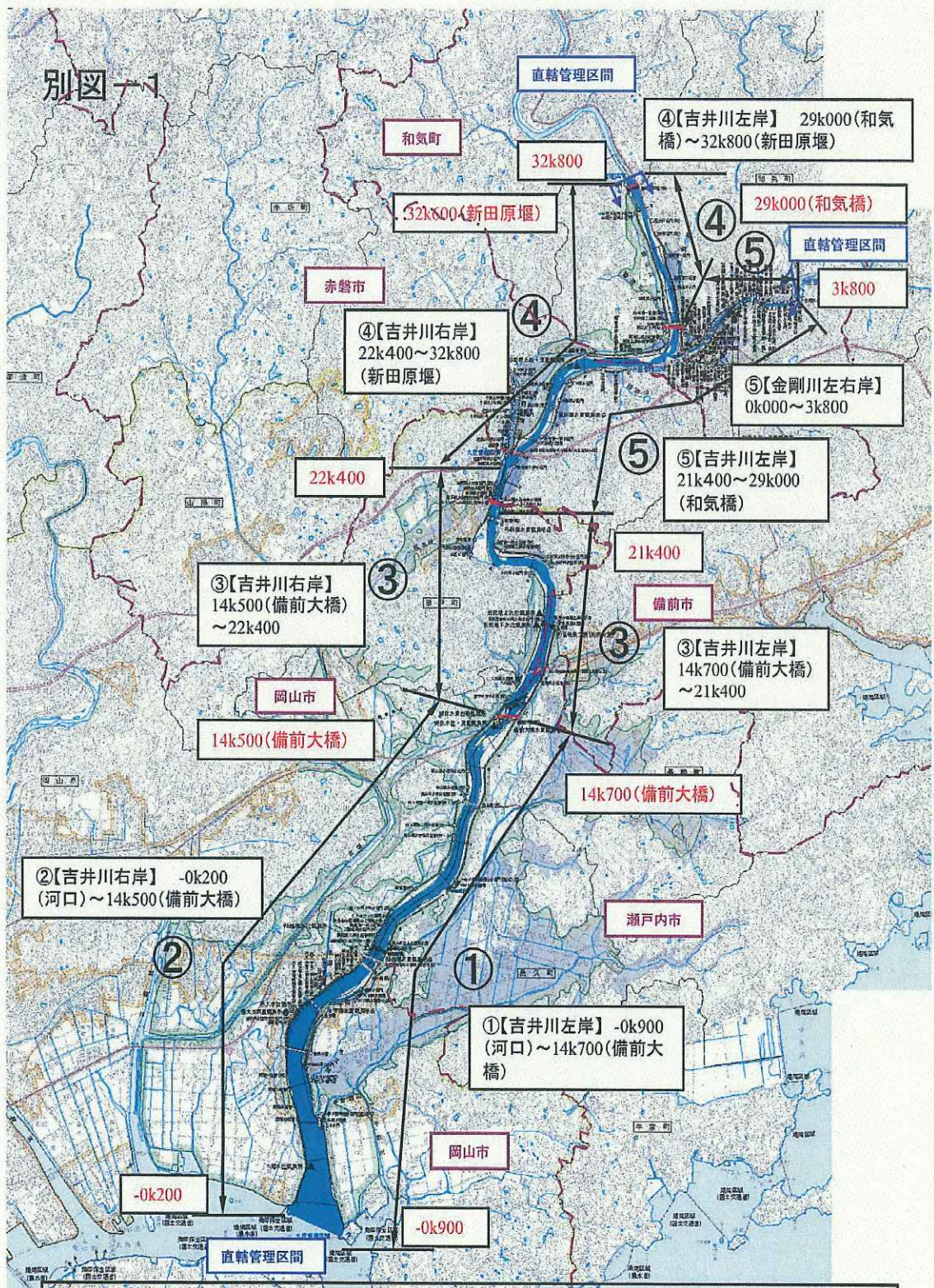
河川等災害応急対策活動等 担当区間図(吉井川)
