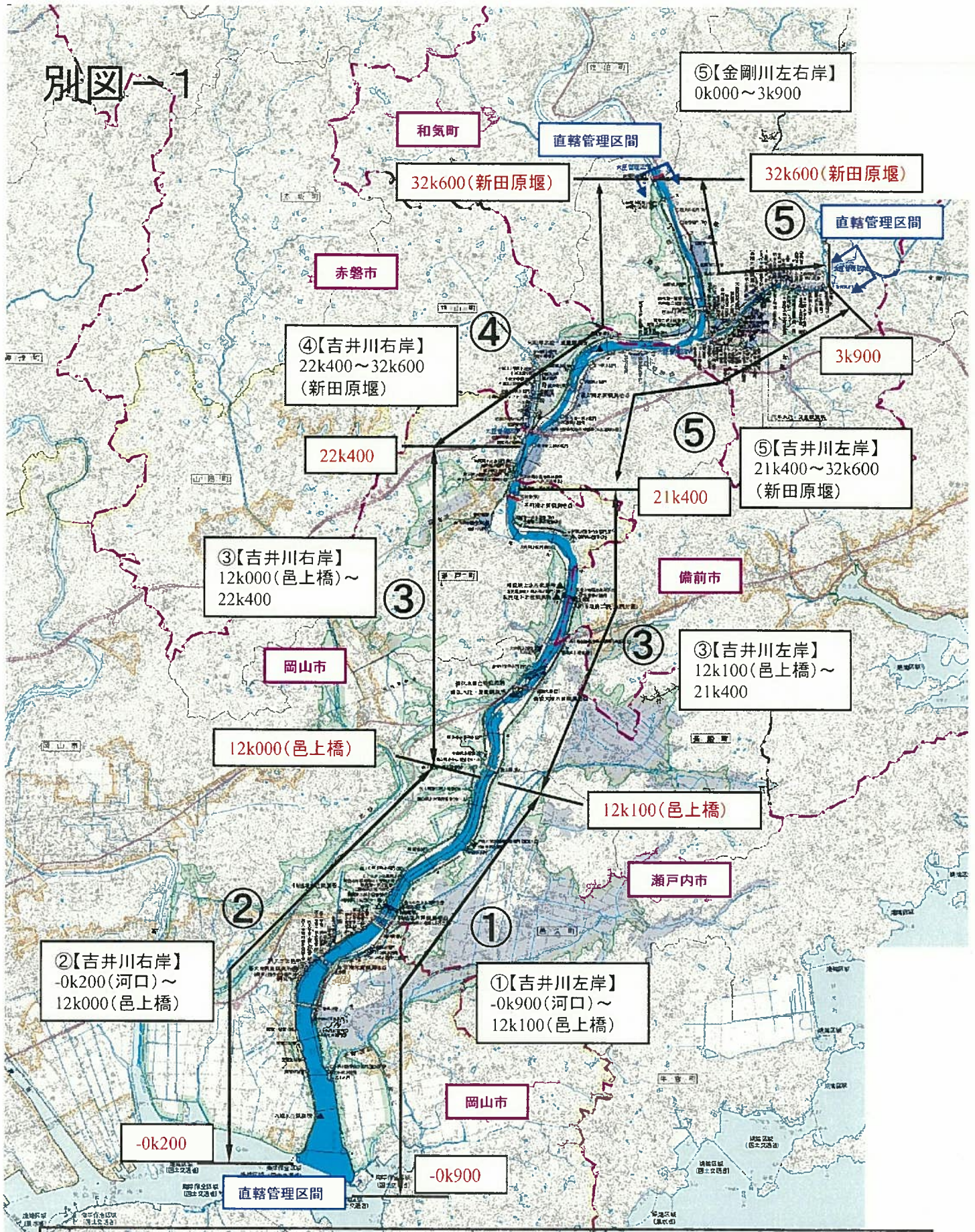
②河川等災害応急対策活動等 担当区間図(吉井川)
