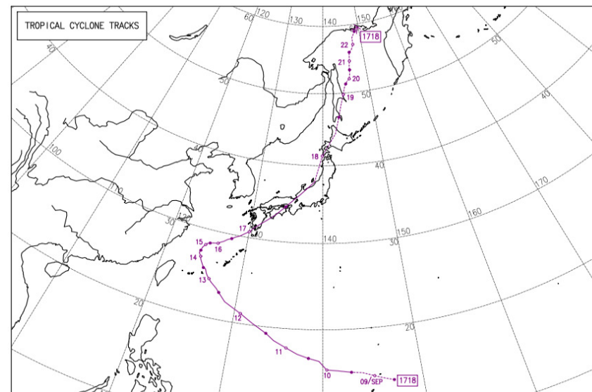
気象庁 台風経路図 平成29年（2017年）台風第18号
