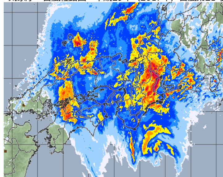
10月22日22時の降水状況（気象庁）
