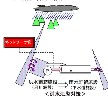
都市水害対策共同事業のイメージ
