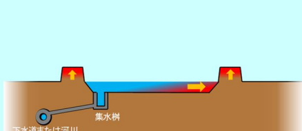
例：調整池の整備・改良
