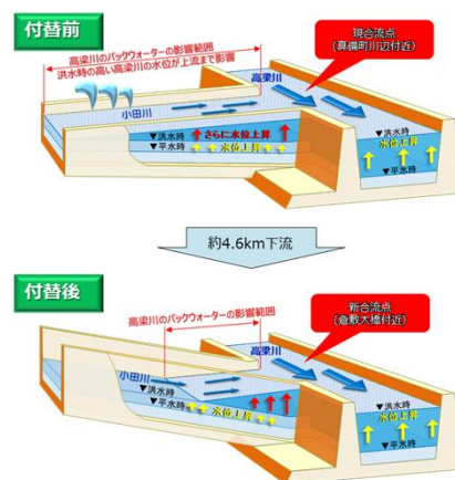
小田川合流点付替えによる整備効果イメージ
