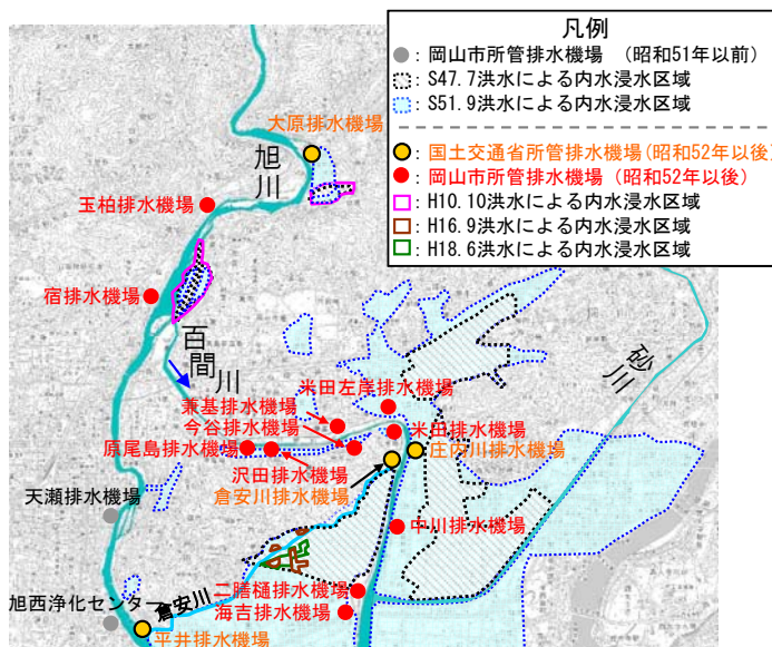
図 3.1.3 過去の主要洪水における内水浸水
