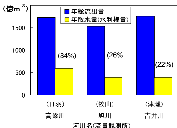
図 3.2.2 岡山県内の一級水系の水利用率
