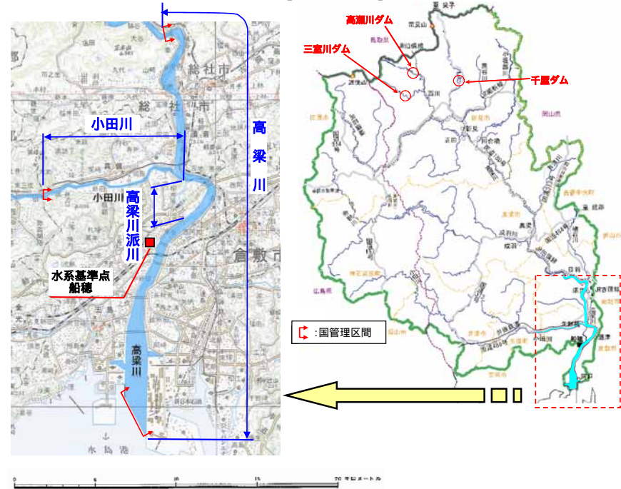
河川整備の計画対象区間の平面図
