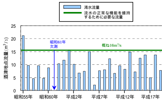
高梁川酒津地点における流況の経年変化
