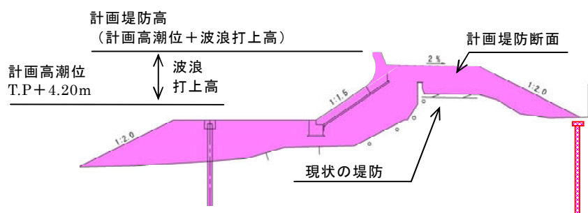
図3.1.12 高潮堤防断面の不足状況(現状堤防と計画堤防との比較)
