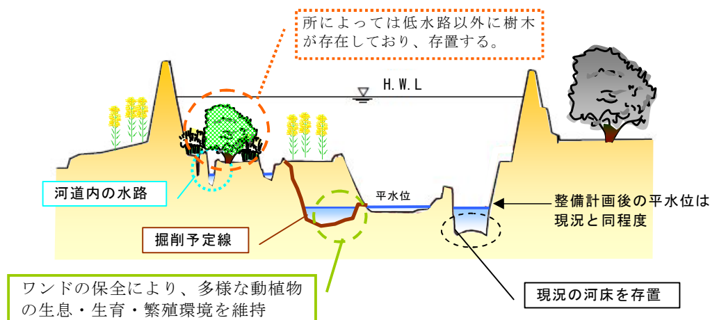
図 5.1.22 ワンド保全のイメージ図
