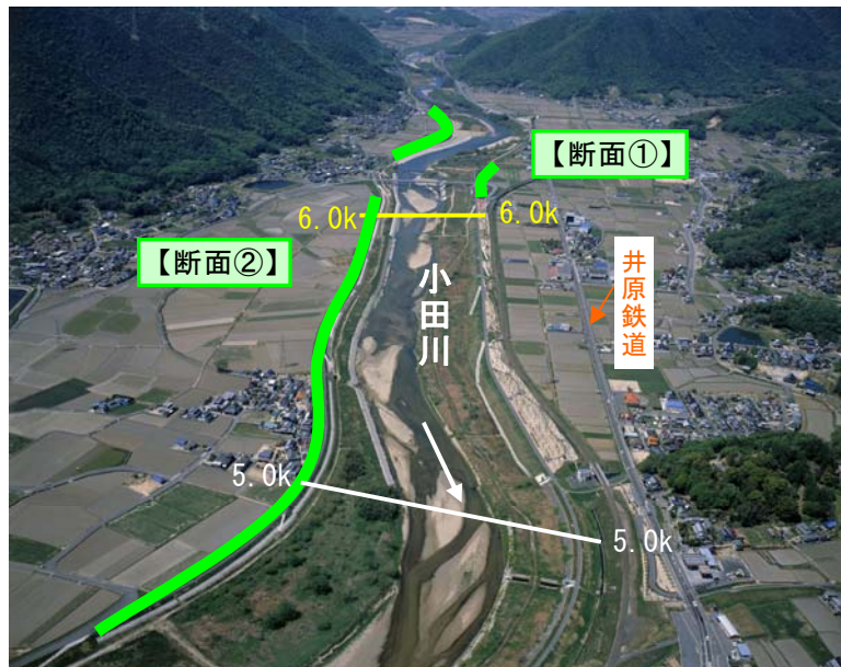
図5.1.29 小田川 築堤（断面確保）の位置図（5.0k～6.0k付近）
