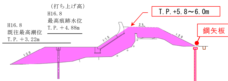
図5.1.4 築堤(高潮堤(耐震対策))のイメージ図(右岸)
