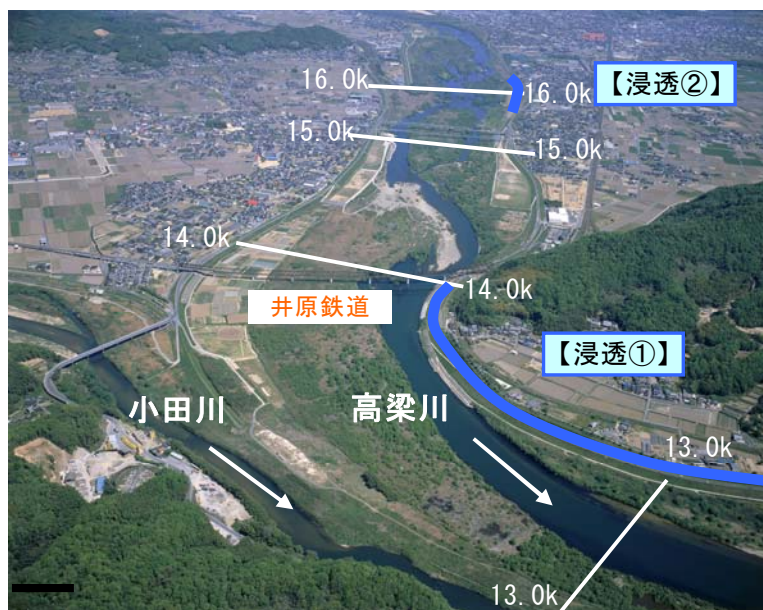
図5.1.18 高粱川 堤防補強（浸透対策）の位置図（13.0k～16.0k付近）
