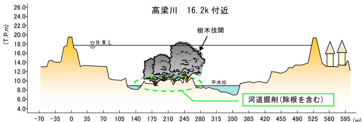
図5.1.16 高粱川 河道掘削及び樹木伐開の位置図(16.0k～17.0k付近)
