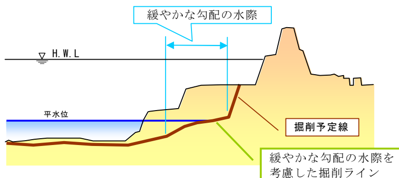
図 5.1.23 緩やかな勾配の水際の保全のイメージ図
