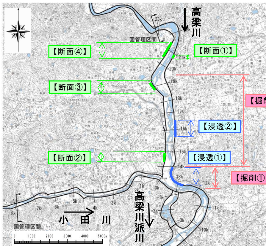
図 5.1.10 河川の整備を実施する区間の位置図(高梁川中流地区(酒津地先～湛井地先))
