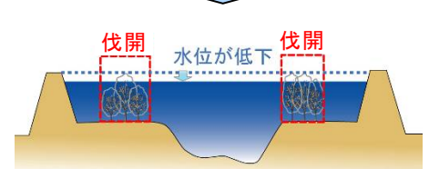
図 5.2.2 樹木伐採による水位低下のイメージ
