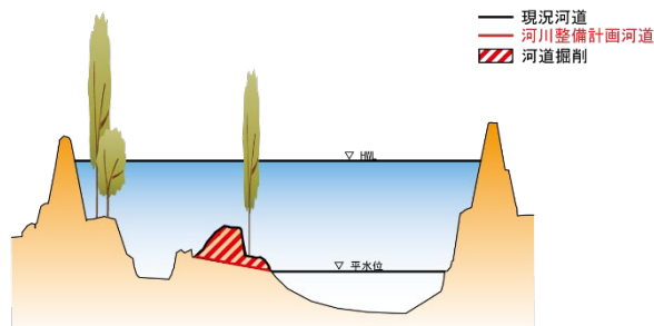
掘削が必要な断面 (21.6k付近)
