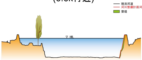
築堤が必要な断面 (6.6k付近)
