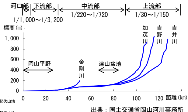
図1.1.3 河床勾配
