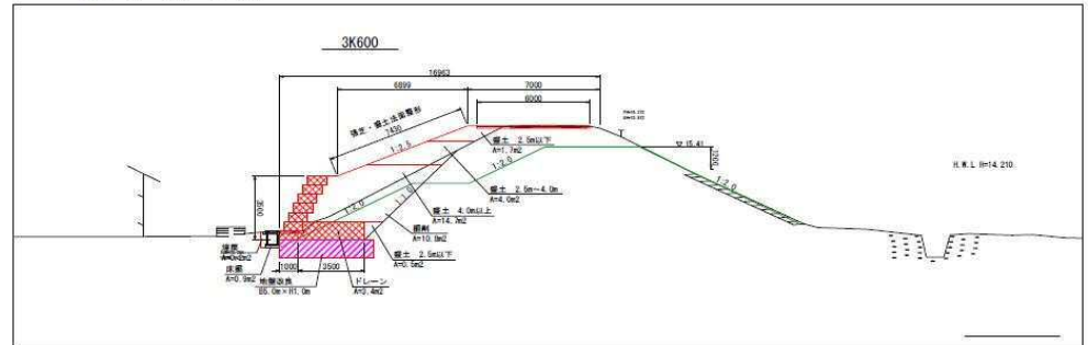
横断図
