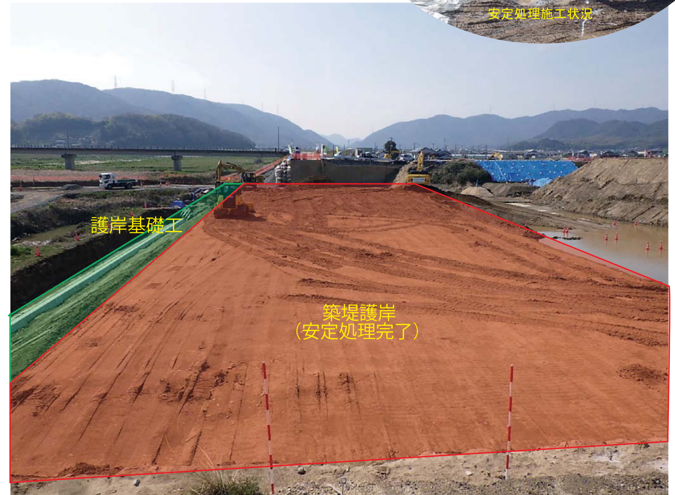
護岸基礎工および築堤護岸底面部改良工（安定処理）施工状況
