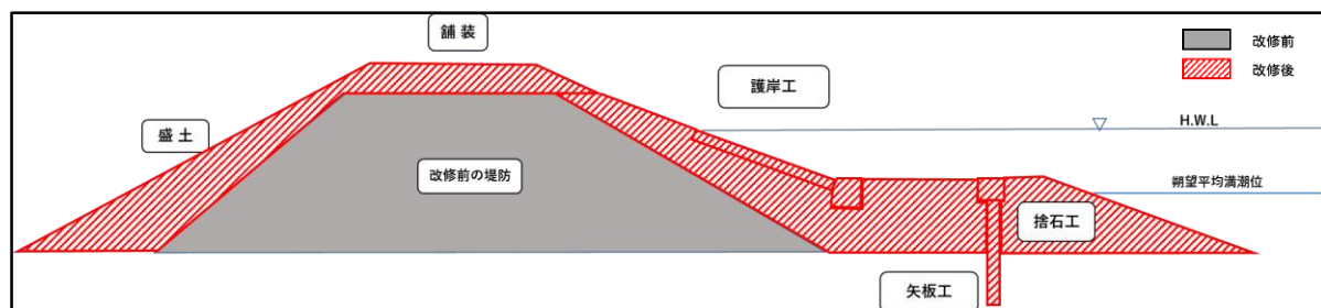
平井地区 整備断面のイメージ図
