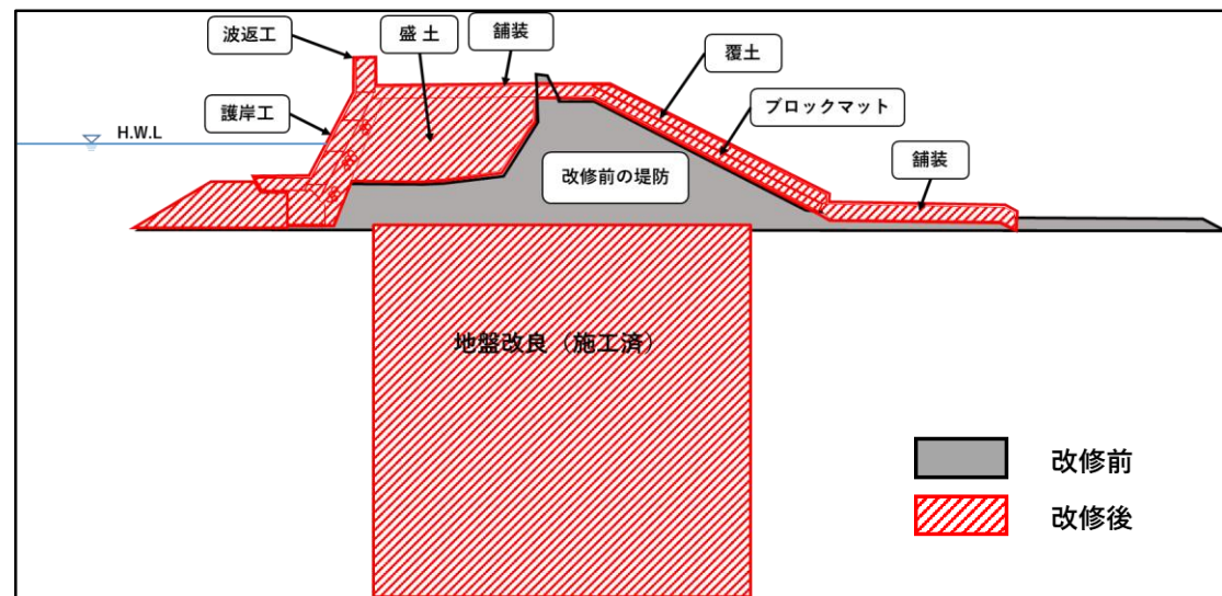
九蟠地区 整備断面のイメージ図
