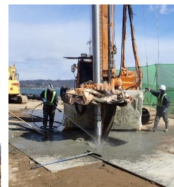
耐震対策の施工状況 (九蟠地区)
