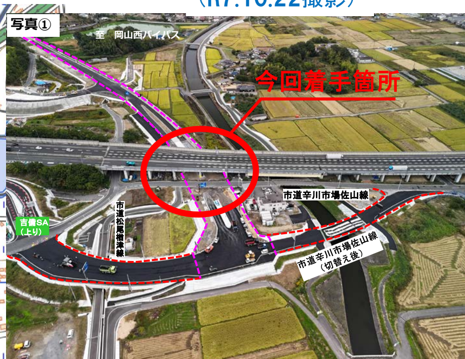
吉備SIC (上り) 付近から終点付近 施工状況
