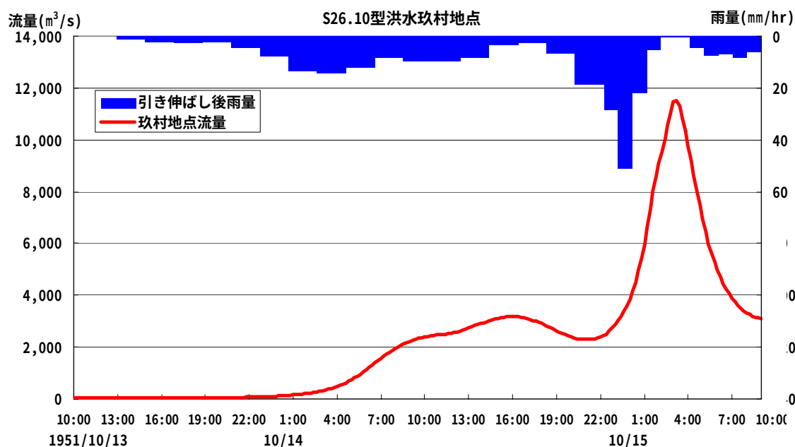
図 4-7 昭和 26 年 10 月型ハイドログラフ(玖村地点)
