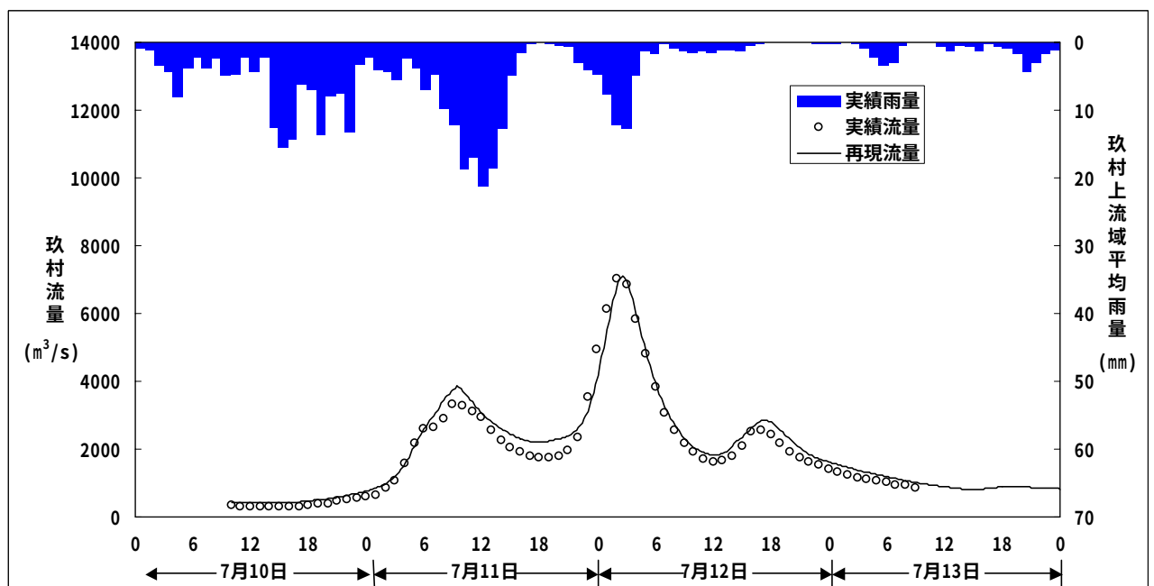
図 4-2 昭和 47 年 7 月洪水再現計算結果(既定計画モデル：玖村地点)
