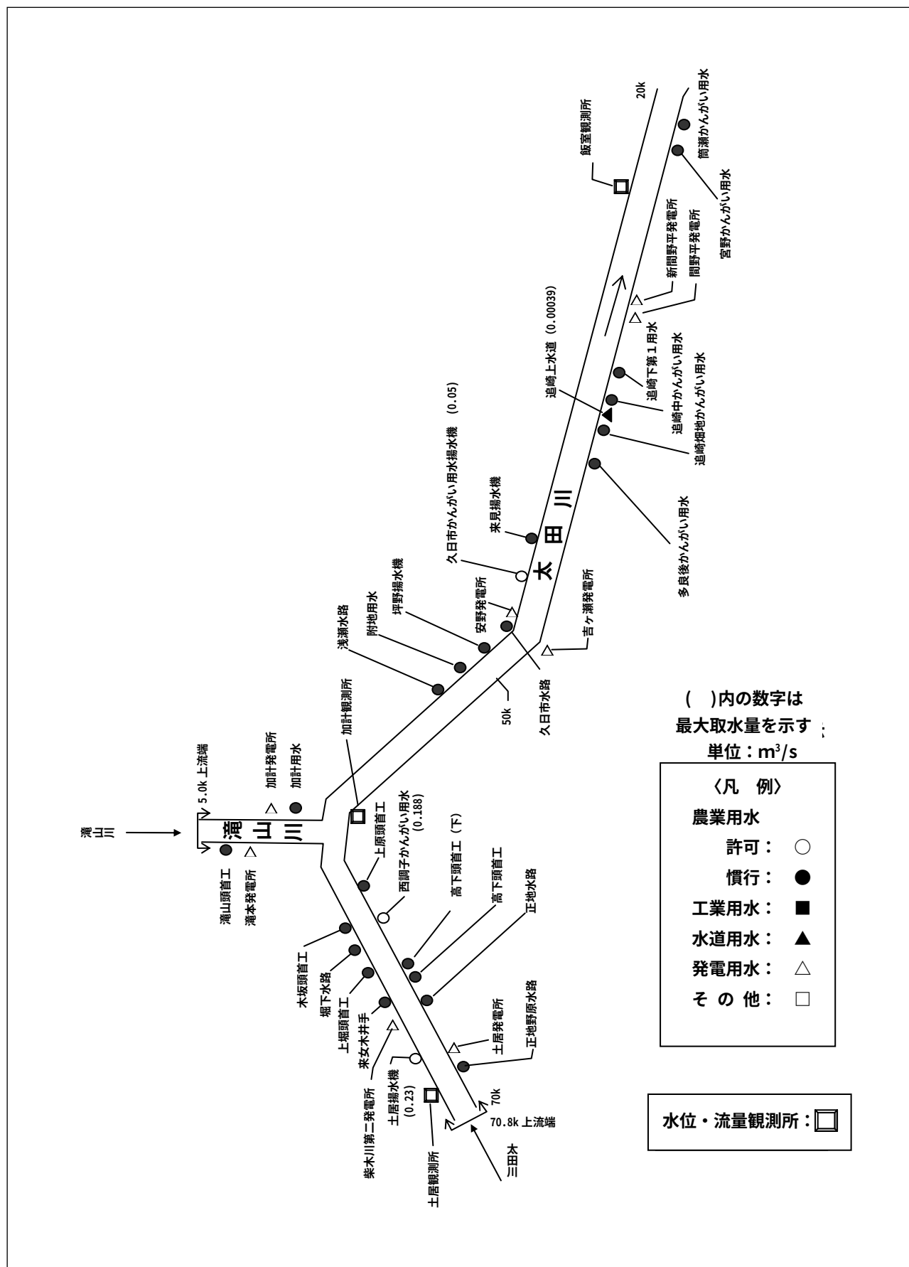
図 2-2 太田川水系の主な水利用状況（上流） 模式図
