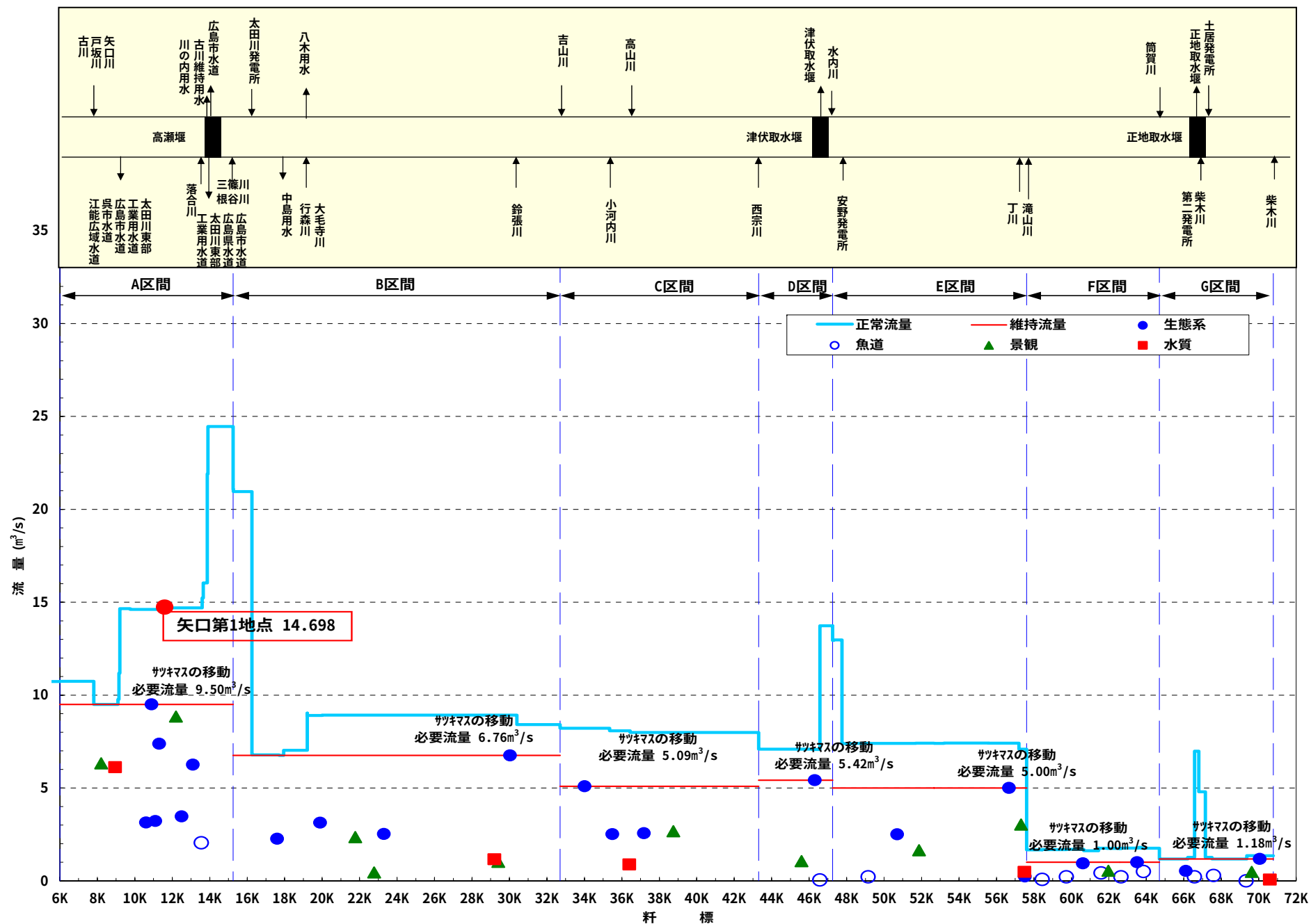
図 6-2(5) 太田川 水収支縦断図 かんがい後期 (6 月 21 日～9 月 30 日)
