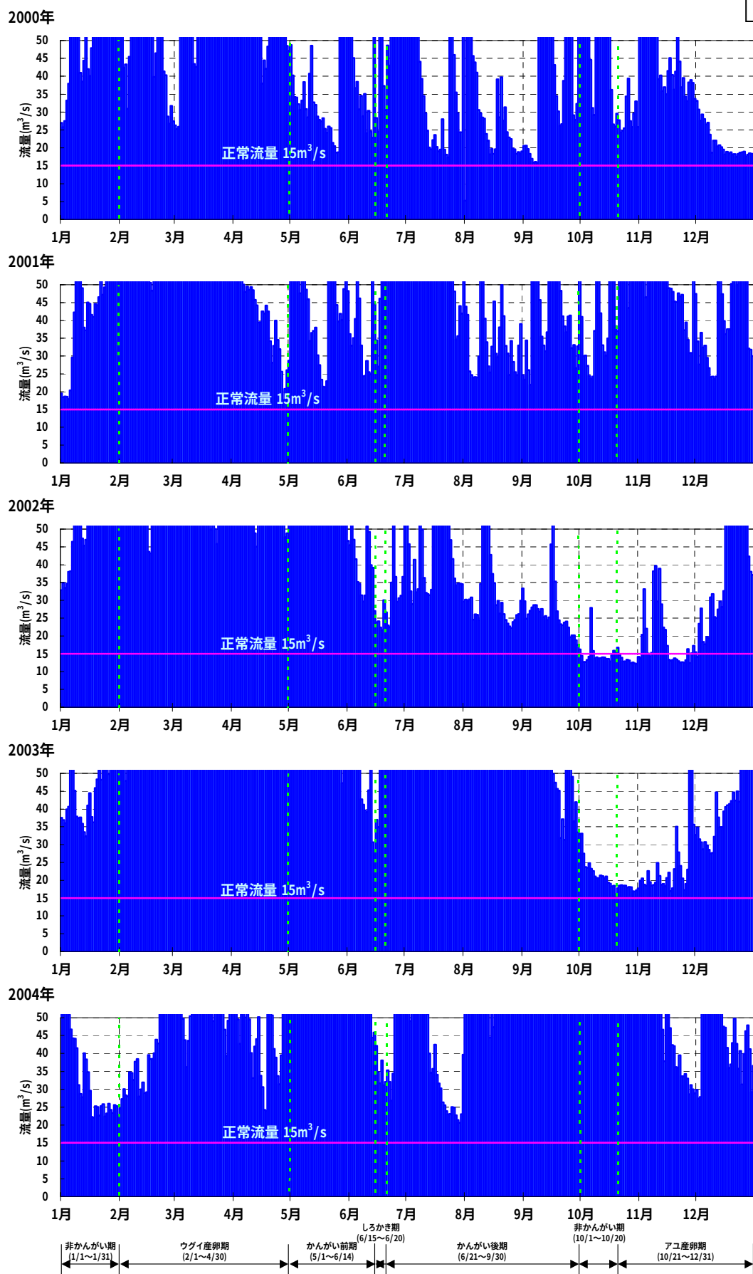
図 6-3(2) 日平均流量図 矢口第 1 地点 (矢口第 1 水位・流量観測所：2000～2004 年)
