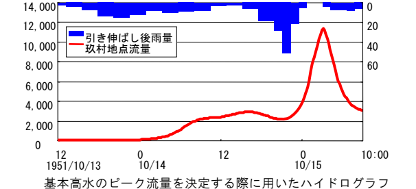
基本高水のピーク流量を決定する際に用いたハイドログラフ
