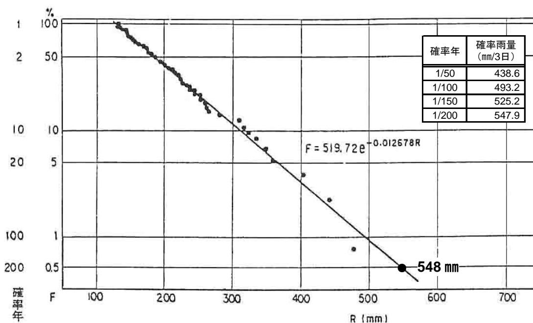
図 4-1 基準地点における雨量確率評価
