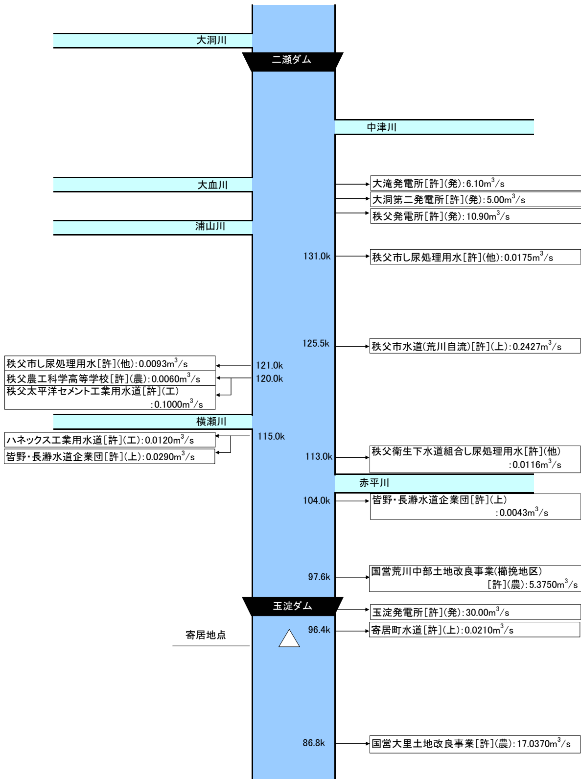
図 2-2 (1) 荒川水系水利模式図
