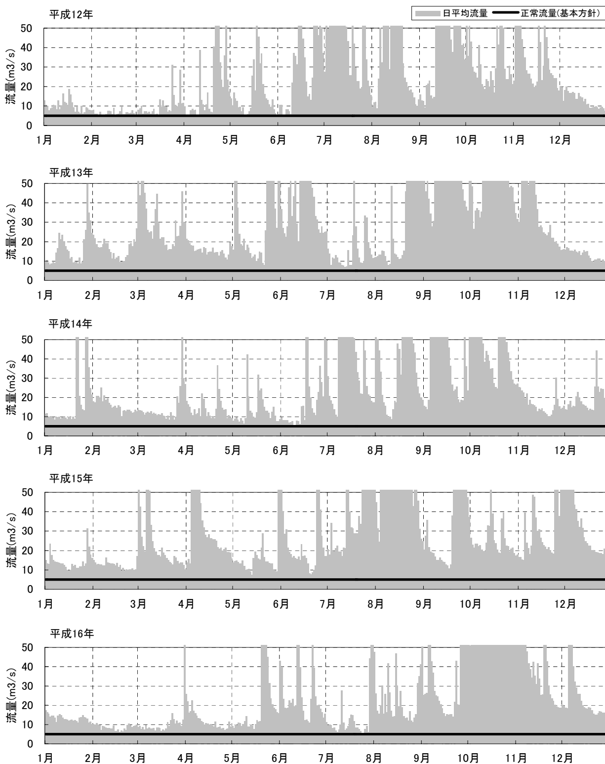
图 6-3 (2) 日平均流量 (秋ヶ瀬取水堰下流地点 : 平成 12 年~平成 16 年)
