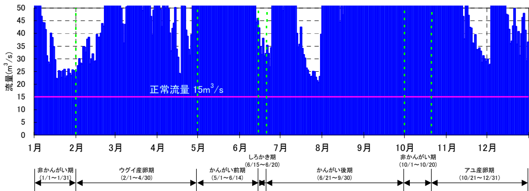
図 6-3 (2) 日平均流量図 矢口第 1 地点 (矢口第 1 水位・流量観測所 : 2000~2004 年)
