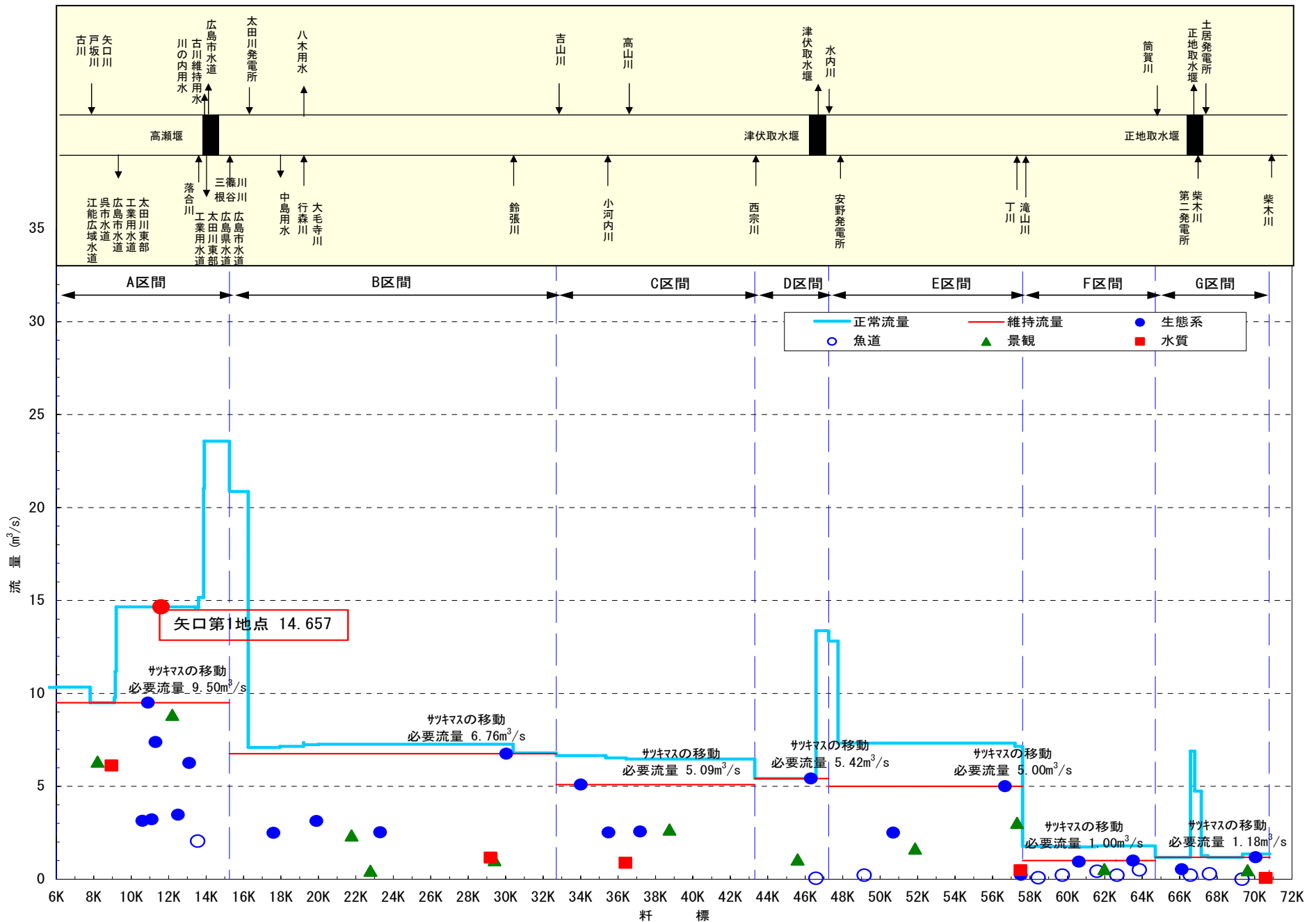
図 6-2(1) 太田川 水収支縦断図 非かんがい期 (1月1日~1月31日)
