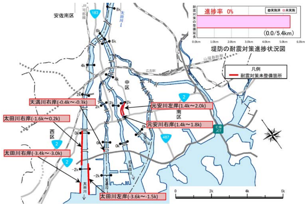
図 3.1.37 耐震対策の整備状況
