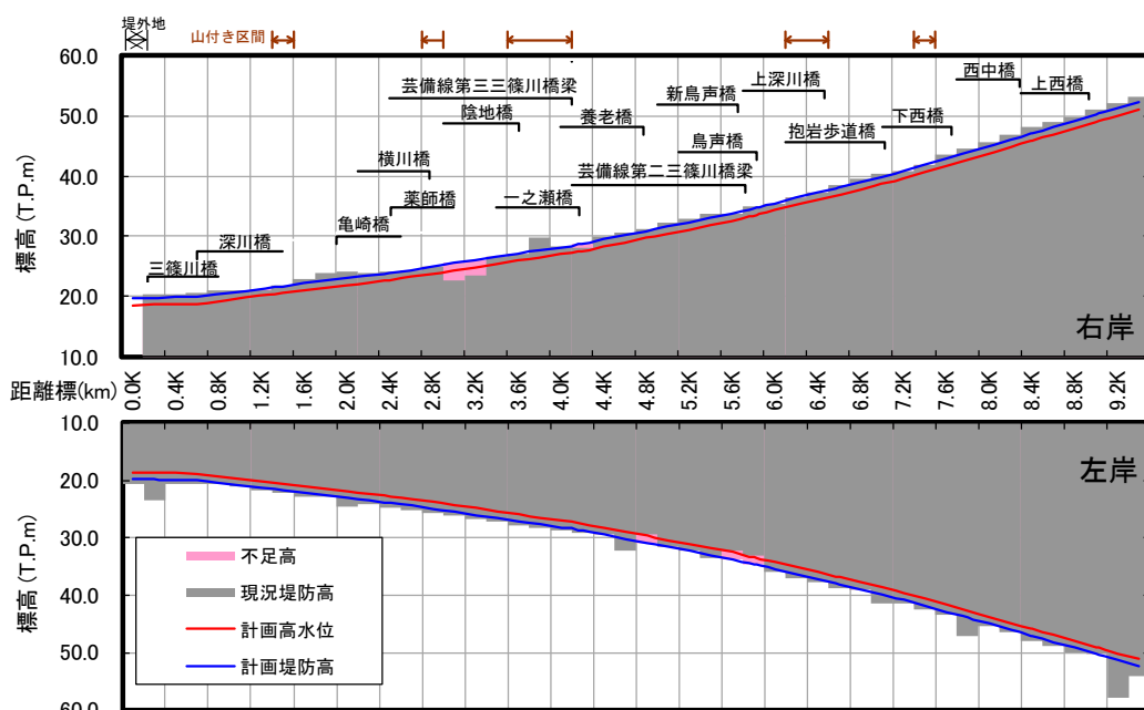
図 3.1.57 堤防高縦断図(三篠川) ※令和2年3月末時点
