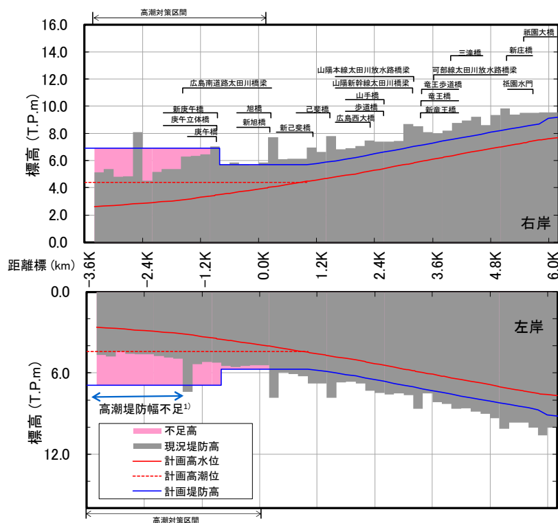
図 3.1.32(1) 堤防高縦断面図(太田川)¹) ※令和2年3月末時点
