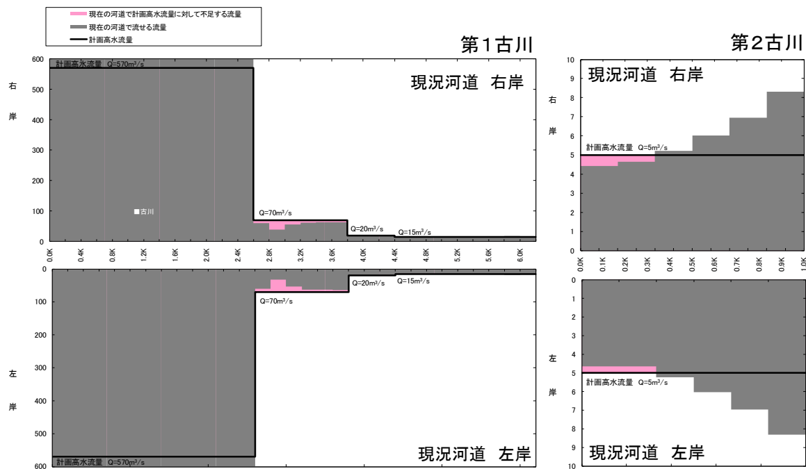
図 3.1.44 現況流下能力図(第1古川、第2古川) ※令和2年3月末時点
