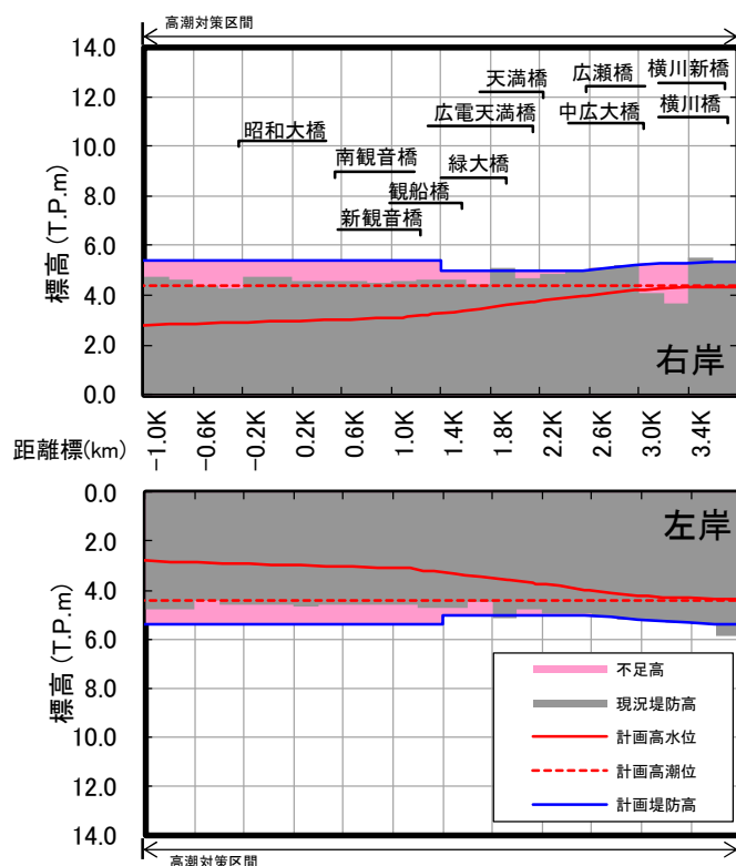
図 3.1.32(2) 堤防高縦断面図(天満川) ※令和2年3月末時点
