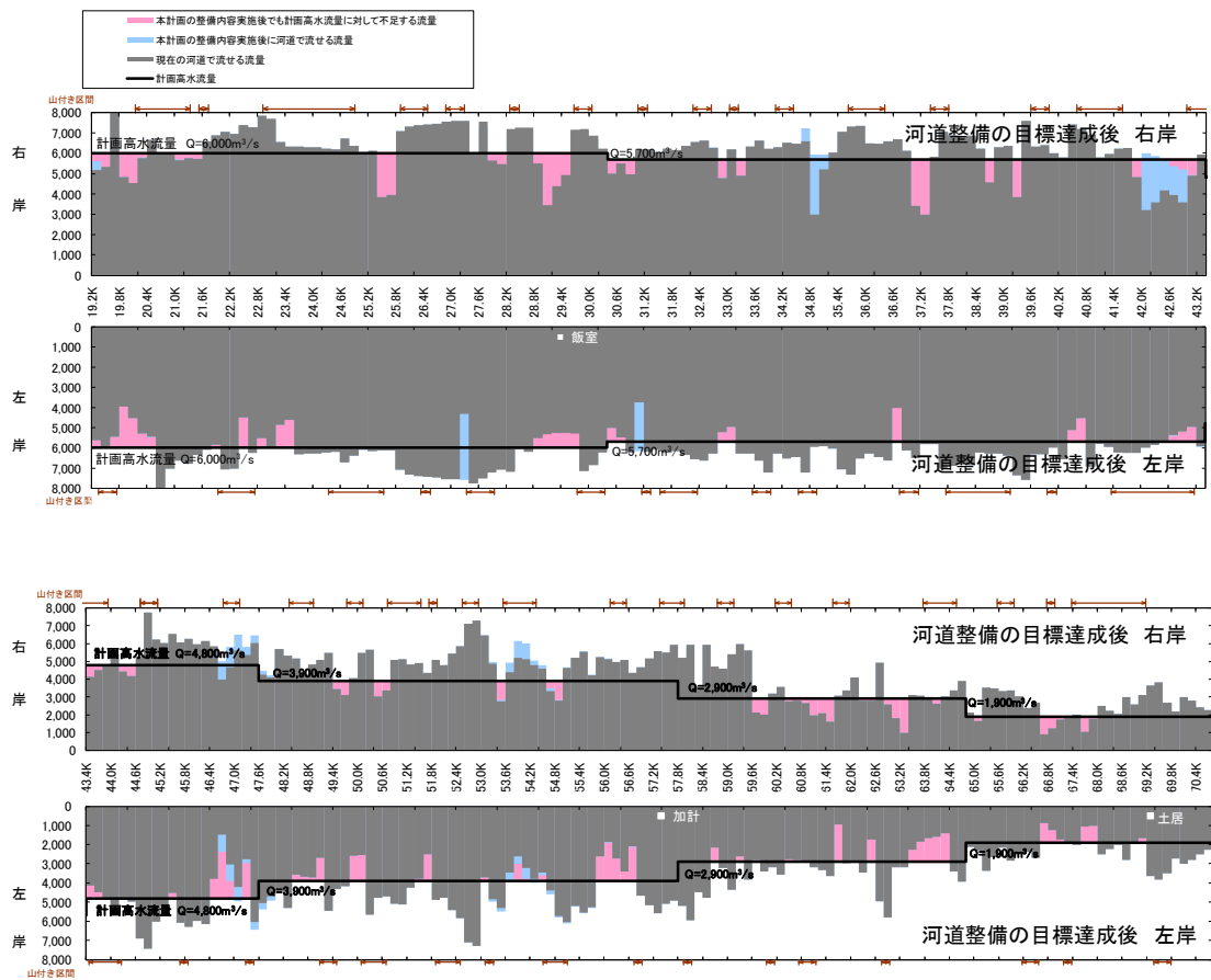
図 5.1.16 流下能力図（中流部）
