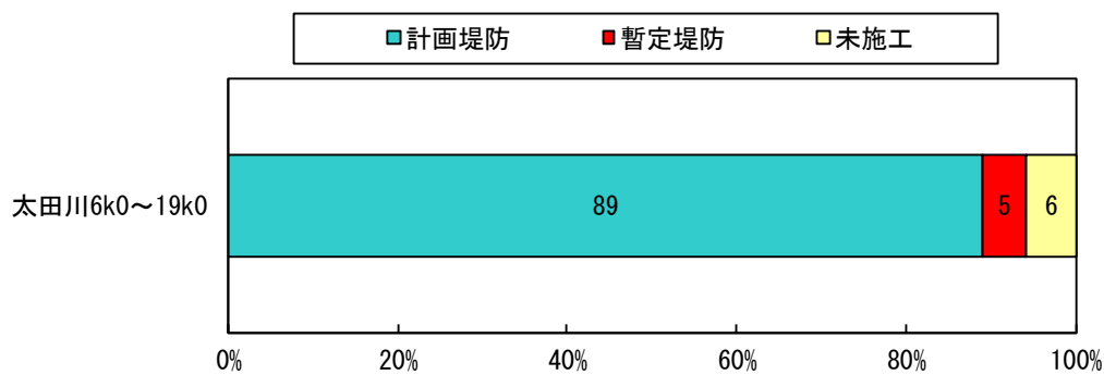
図 3.1.43 堤防整備率(下流部) ※令和2年3月末時点
