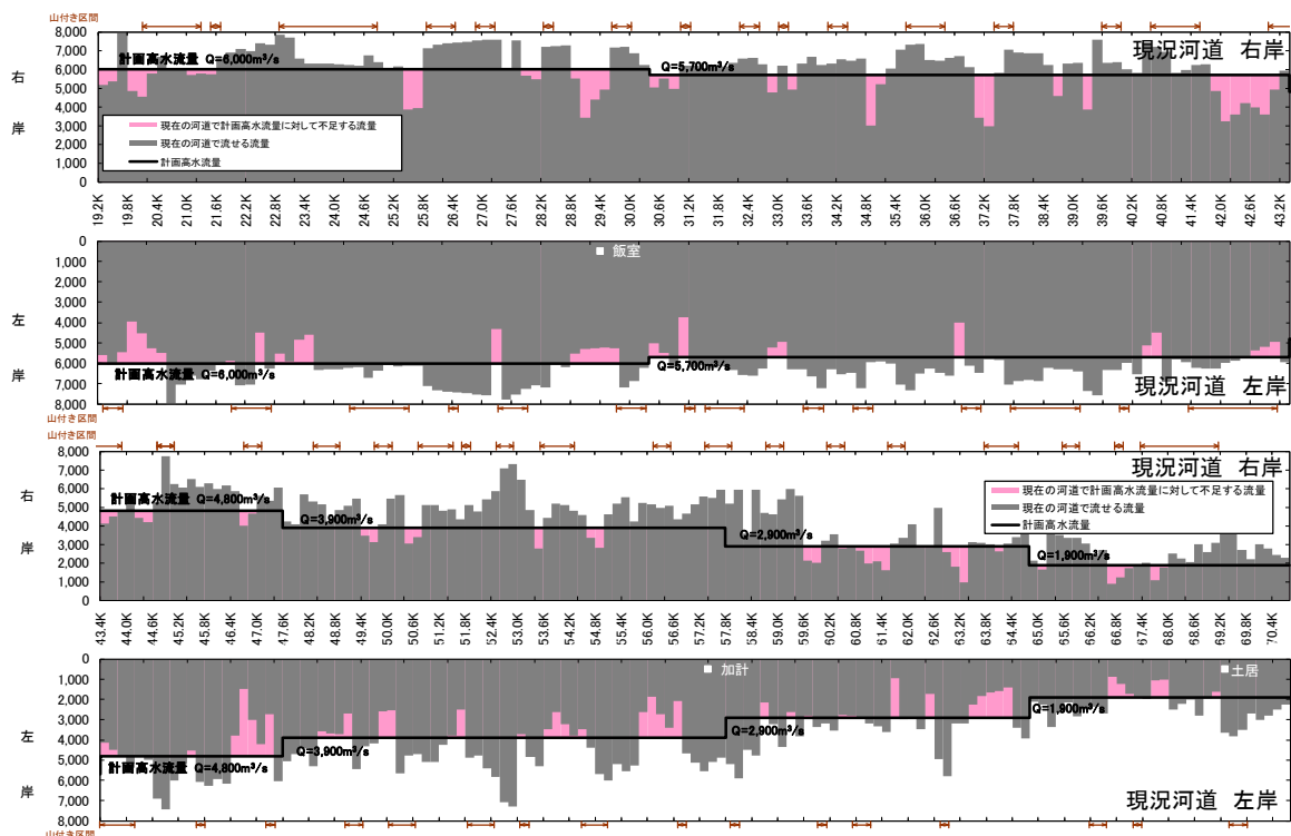
図 3.1.50 現況流下能力図(中流部)
