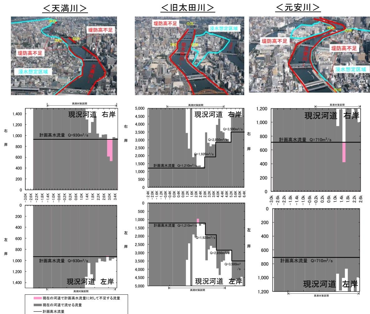
図 3.1.31 現況流下能力図(市内派川)
