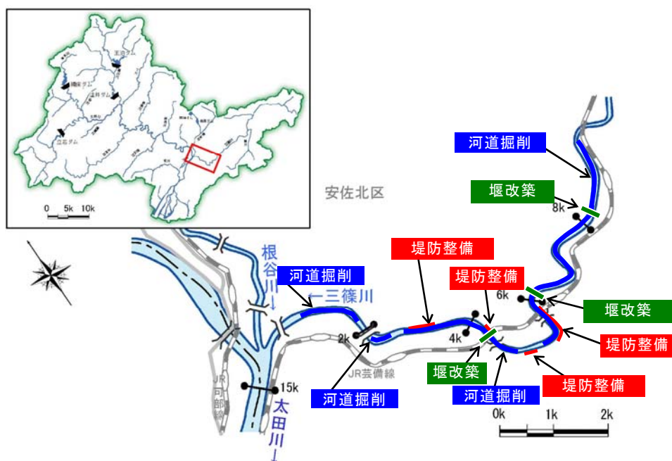
図 5.1.19 洪水対策の整備箇所位置図（三篠川）
