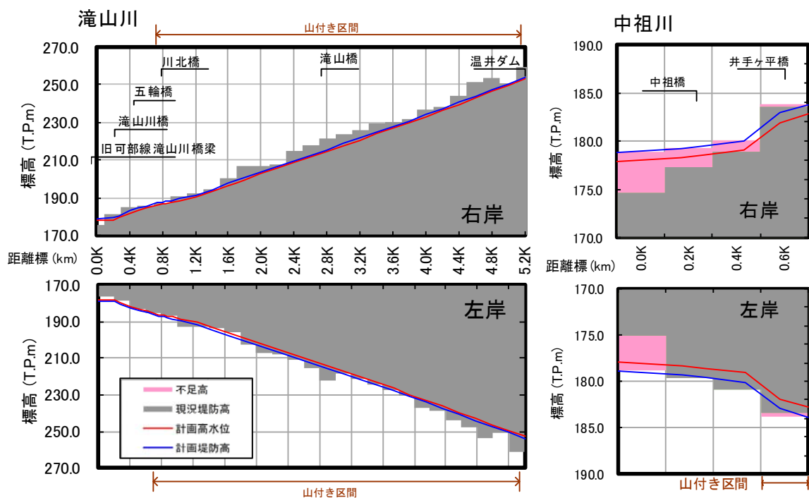
図 3.1.67 堤防高縦断面図(滝山川、中祖川) ※令和2年3月末時点
