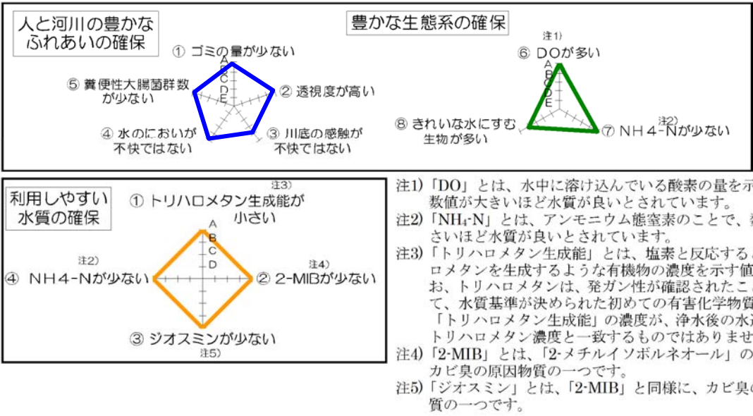
図 3.2.8 太田川水系における「新しい水質指標」の調査結果例
