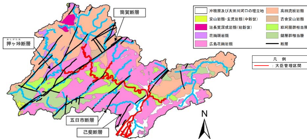
図 2.1.2 太田川流域の地質図
