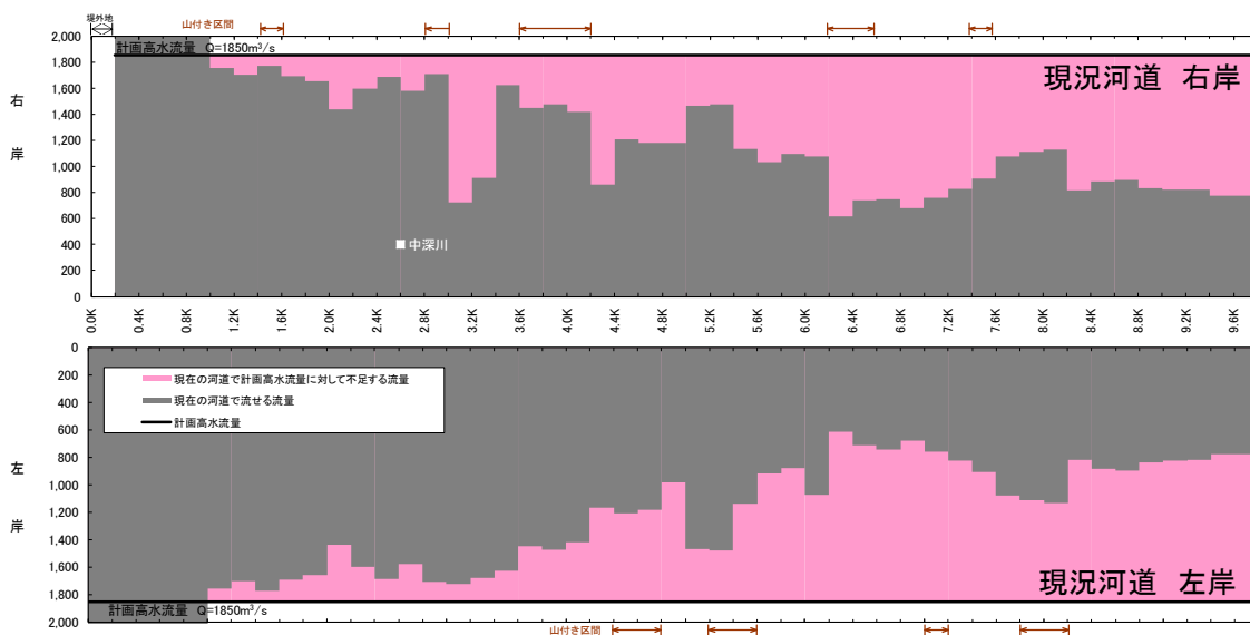
図 3.1.56 現況流下能力図(三篠川) ※令和2年3月末時点
