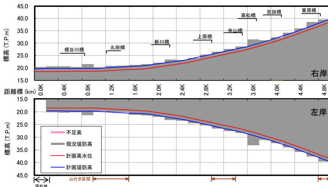
図 3.1.62 堤防高縦断面図(根谷川) ※令和2年3月末時点
