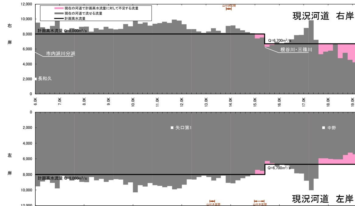
図 3.1.41 現況流下能力図(下流部)
