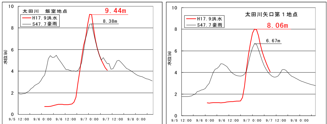
図 3.1.9 飯室水位・流量観測所及び矢口第1水位・流量観測所の水位
