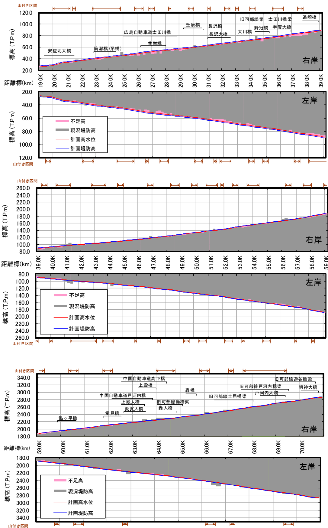
図 3.1.52 堤防高縦断図(中流部)
