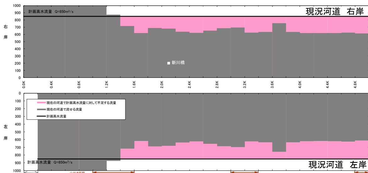
図 3.1.61 現況流下能力図(根谷川) ※令和2年3月末時点
