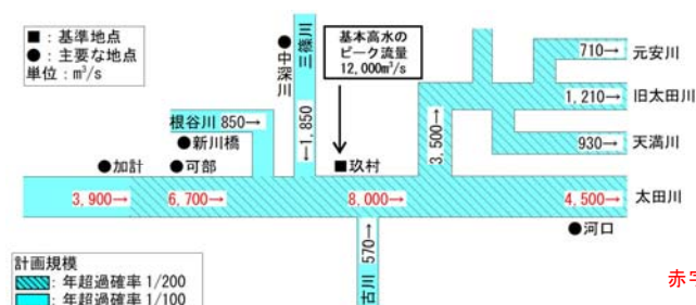
図 2.2.4 工事实施基本計画と河川整備基本方針の流量配分
