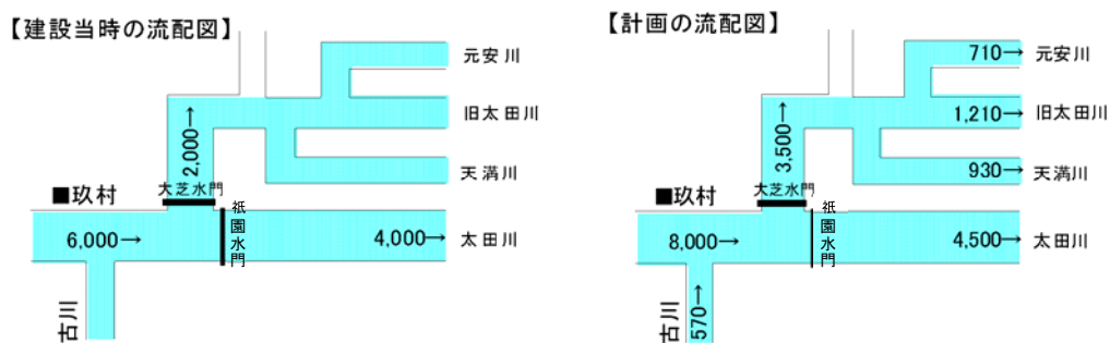
図 3.1.28 流量配分図
