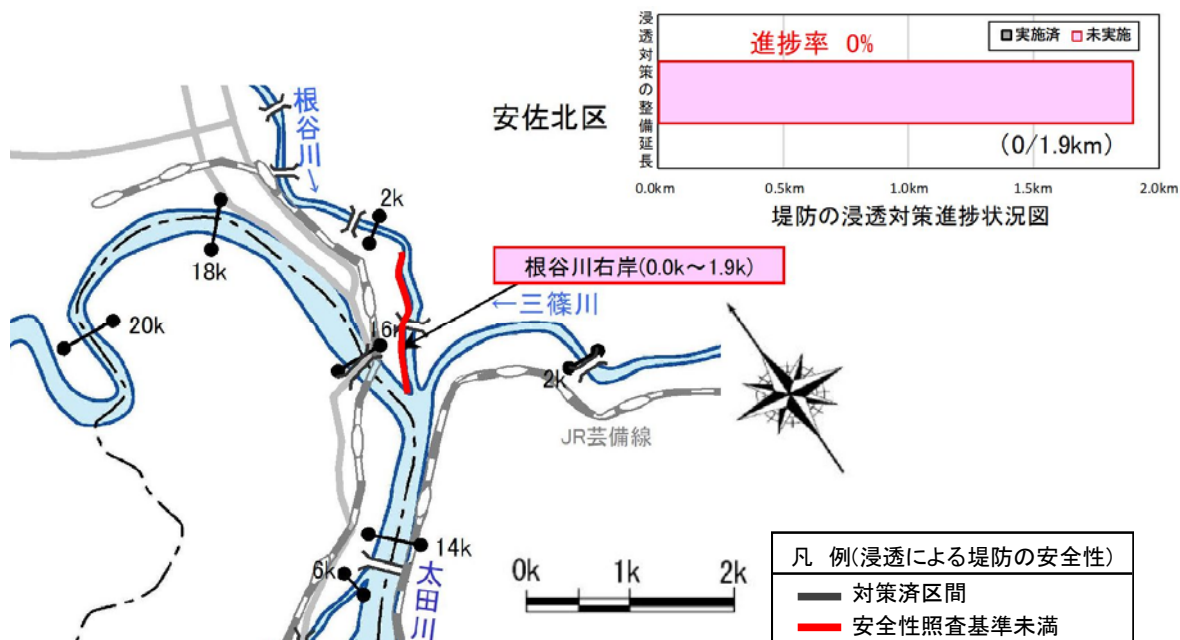
図 3.1.64 堤防の浸透に対する安全性の状況（根谷川）
