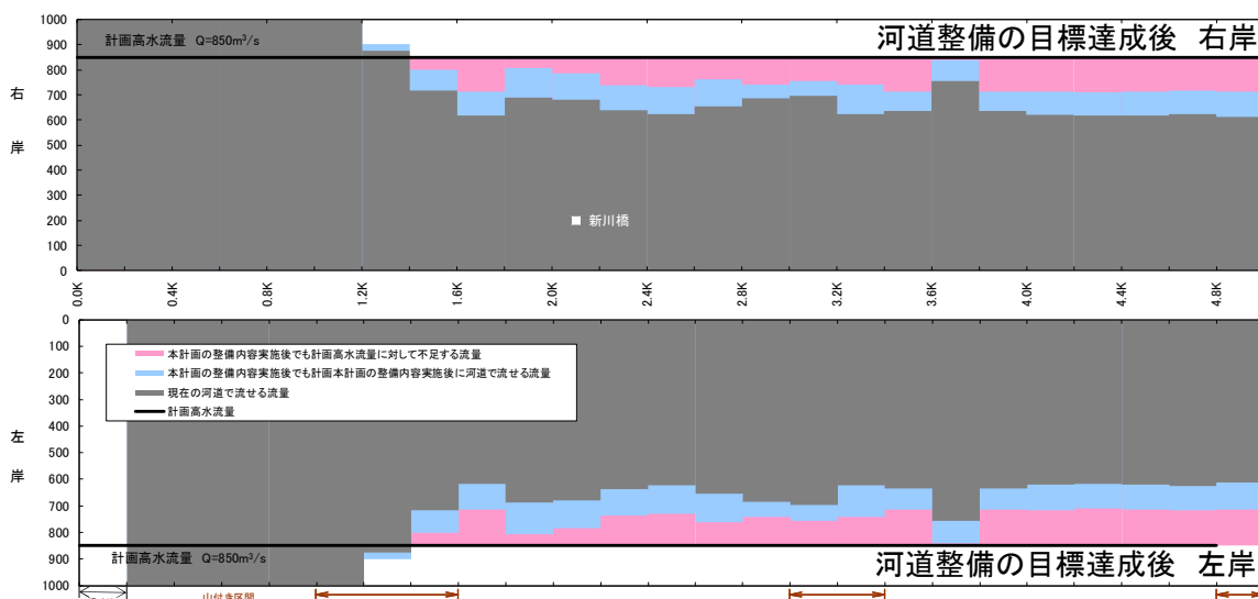
図 5.1.25 流下能力図 (根谷川)
