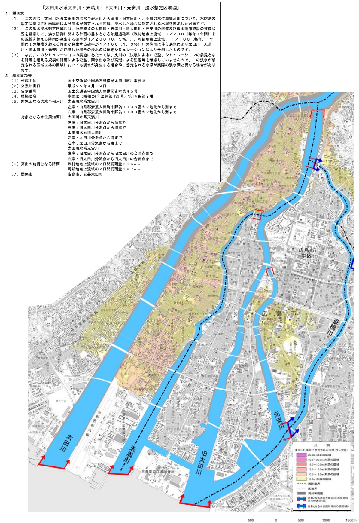
図 3.1.29 現状で計画規模の洪水が発生した場合に浸水するおそれがある範囲
