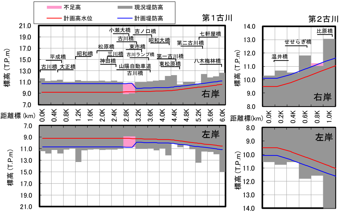
図 3.1.45 堤防高縦断図(第1古川、第2古川) ※令和2年3月末時点
