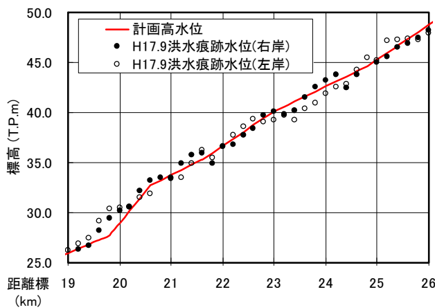
図 3.1.10 中流部における痕跡水位
