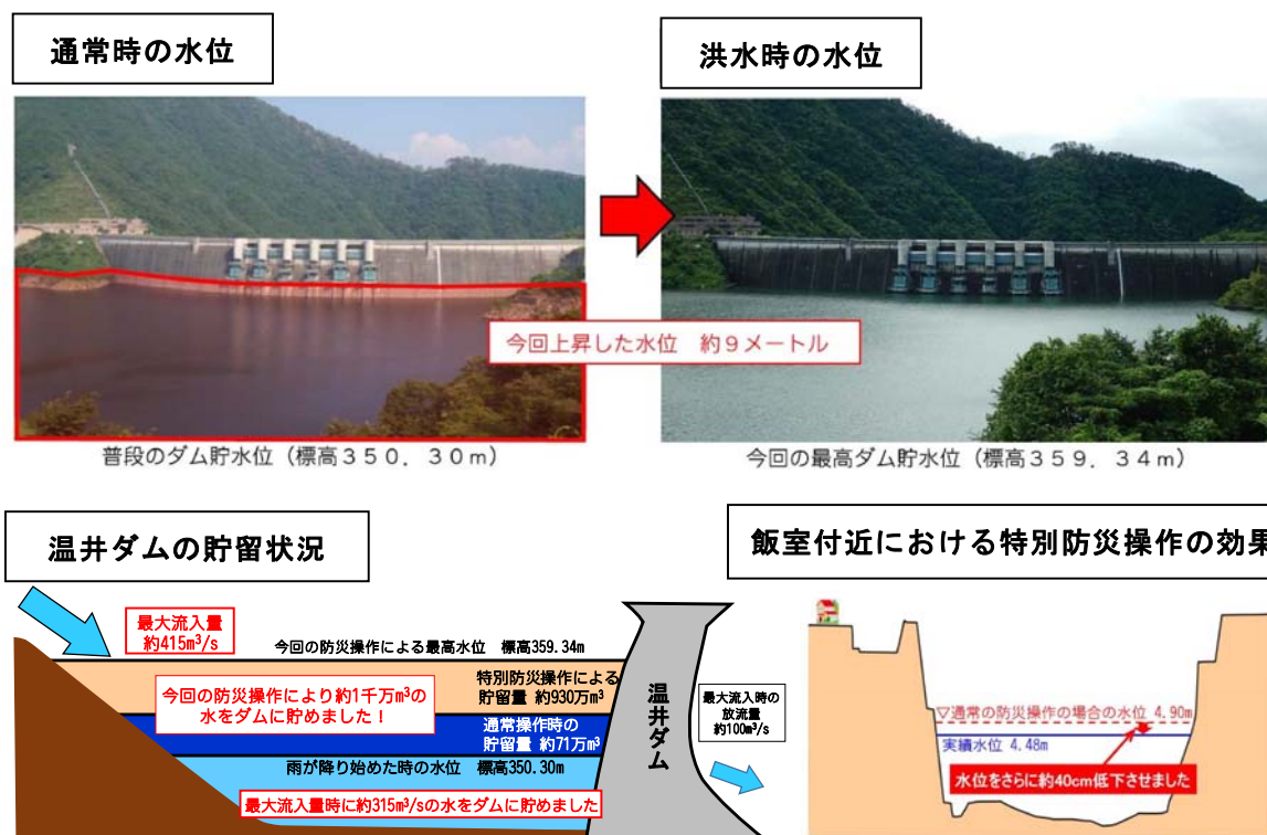
図 3.1.69 平成 30 年 7 月豪雨における温井ダムの洪水調節効果
