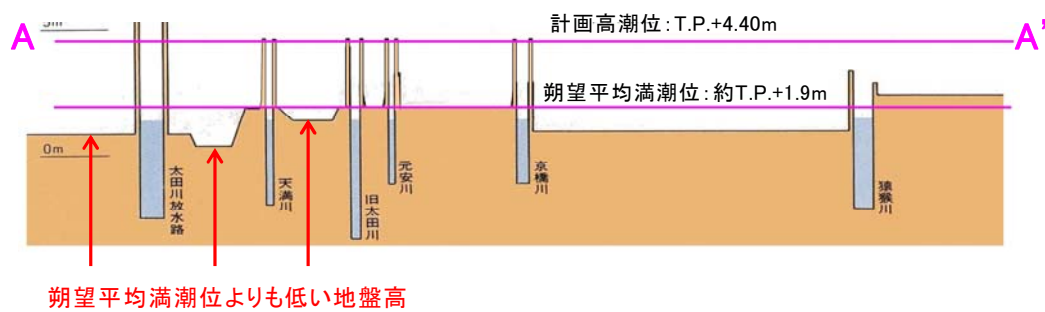
図 3.1.35 下流デルタ域の横断面図
