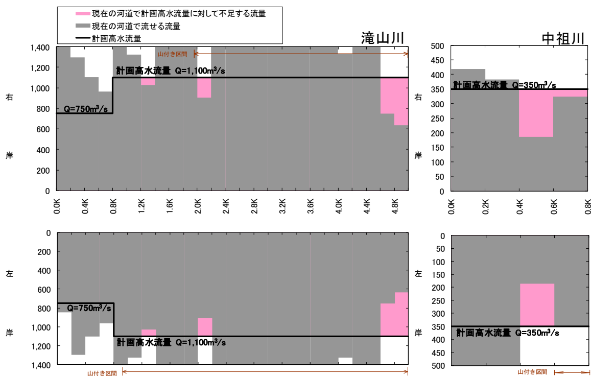
図 3.1.66 現況流下能力図（滝山川、中祖川） ※令和 2 年 3 月末時点
