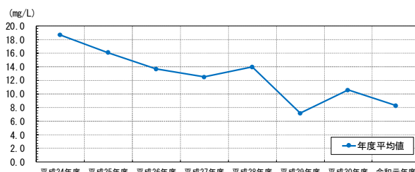
旭橋地点のケイ酸測定値の経年変化 (平成24年度～令和元年度)
