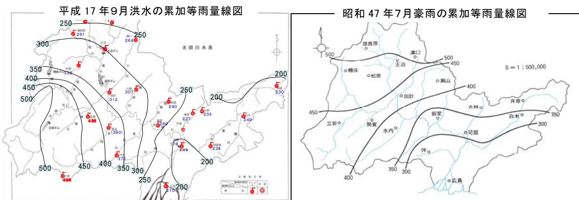
図 3.1.7 等雨量線図
