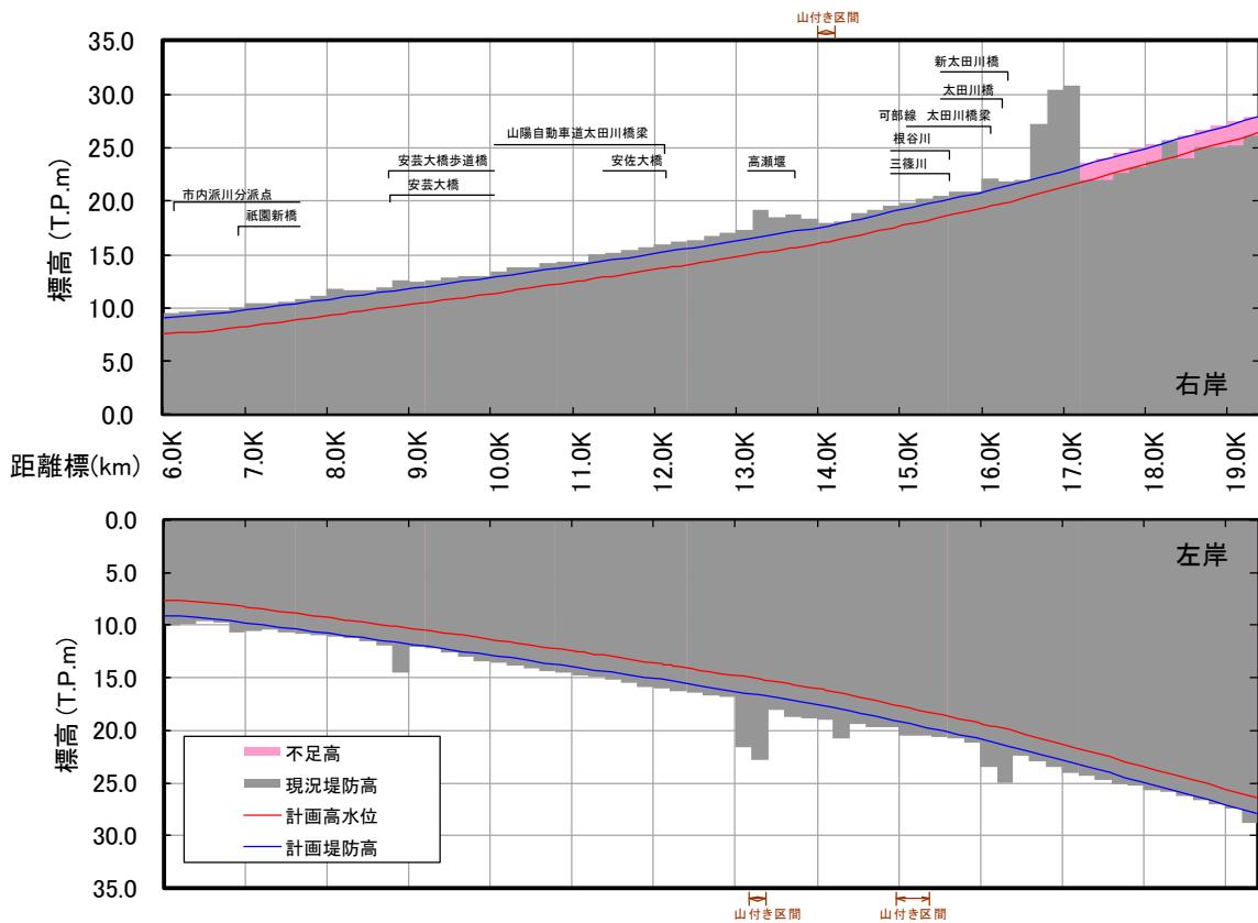
図 3.1.42 堤防高縦断面図(下流部) ※令和2年3月末時点
