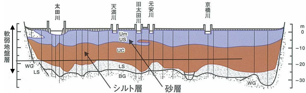
図 3.1.36 下流デルタ域の地質断面図 (A-A' 断面付近)
