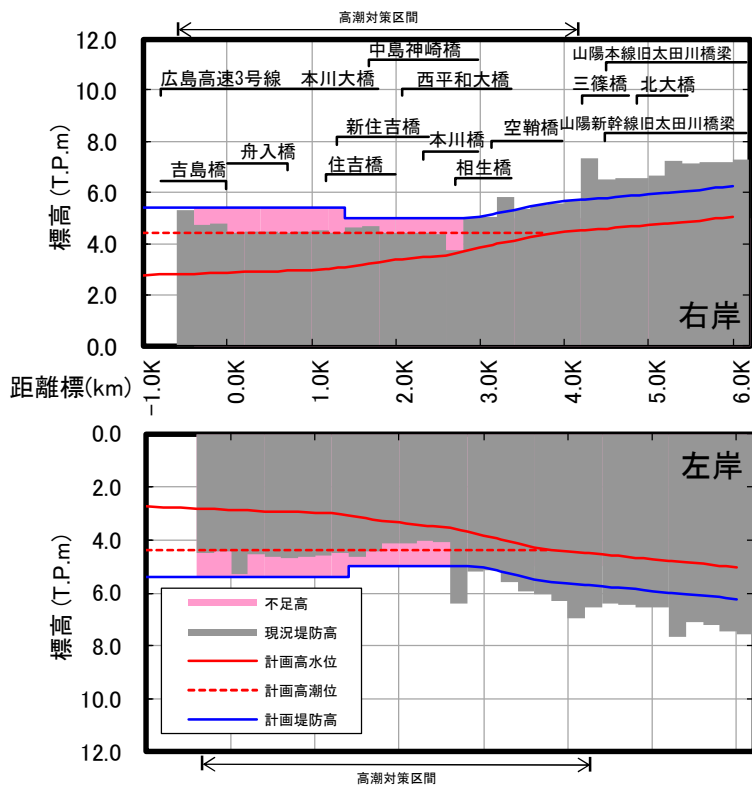
図 3.1.32 (3) 堤防高縦断面図(旧太田川) ※令和2年3月末時点
