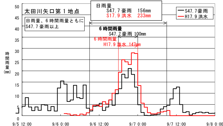
図 3.1.8 矢口第 1 地点流域平均雨量ハイトグラフ
