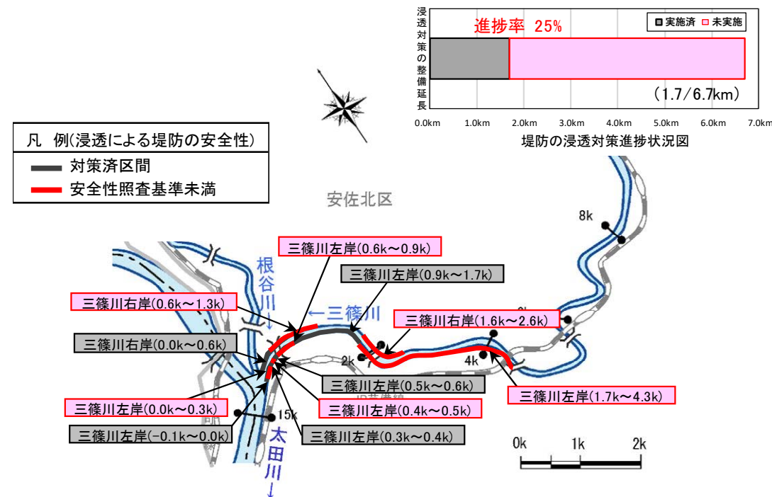
図 3.1.59 堤防の浸透に対する安全性の状況（三篠川）※令和2年3月末時点
