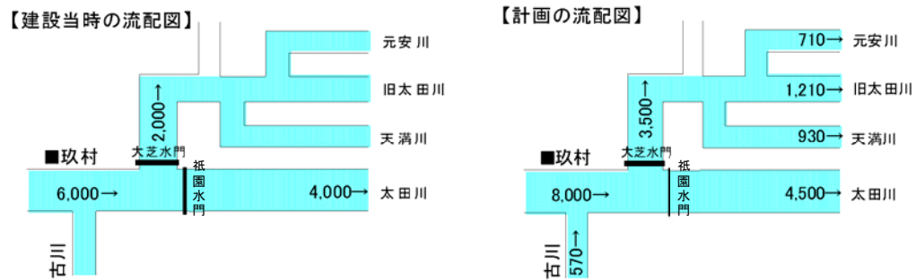
图 3.1.26 流量配分图
