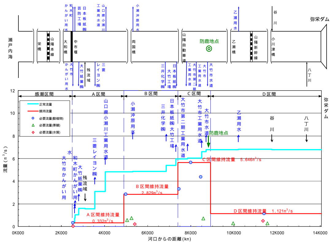
図 6-2(3) 小瀬川 水収支縦断図 (しらかき期 : 5/10 ~ 6/11)
