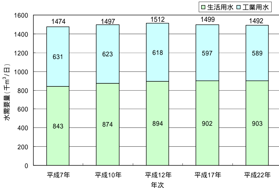
図 3-1 広島県長期水需給計画(広島地域)
