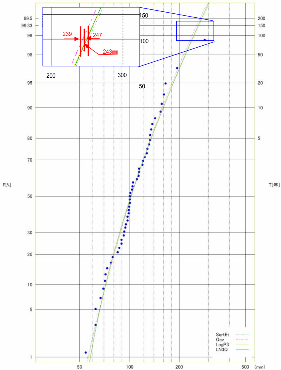
図 4- 5 両国橋地点 確率雨量評価 (S30 ~ H17, 51 ヶ年)
