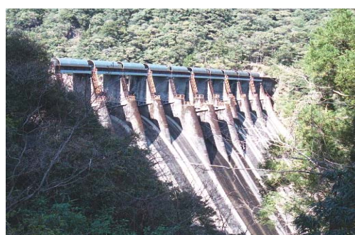
松尾ダム
