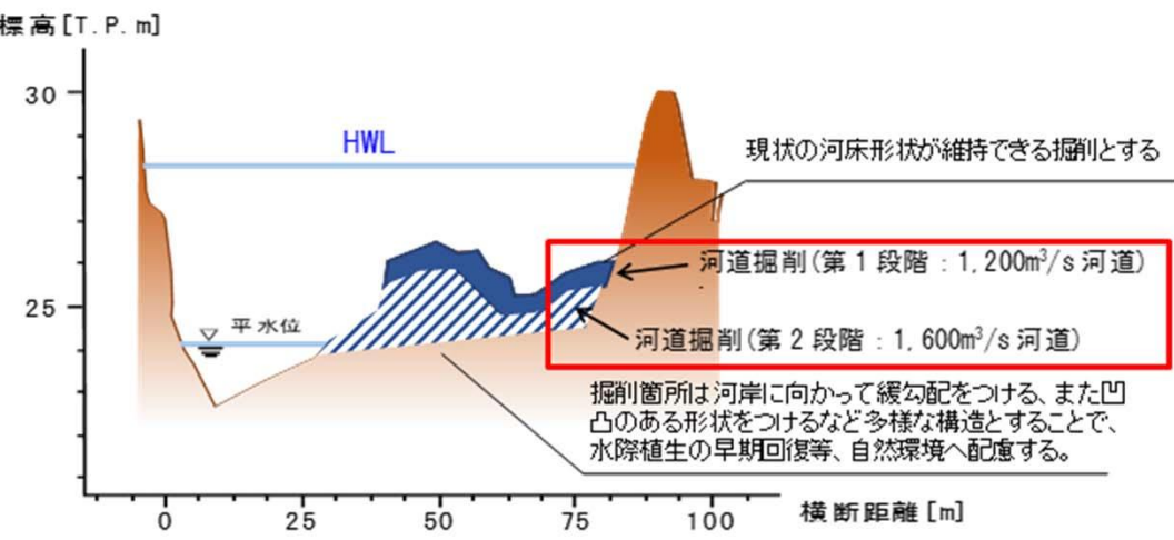
横断面図
