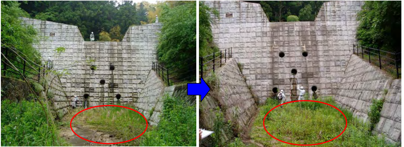
昨年度と比べて、流路工の堆積土砂はありませんでした。また、コンクリートのひび割れは確認されませんでした。(四季が丘6号砂防えん堤下流部)
