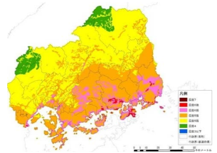
南海トラフ巨大地震
