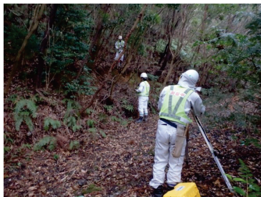
測量作業状況
