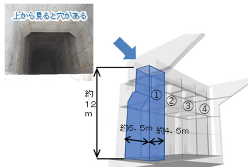
栗野川橋下部工 3Dモデル
