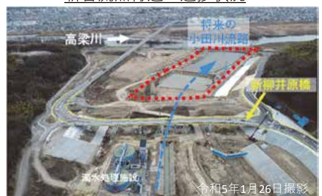
新合流点付近の進捗状況
