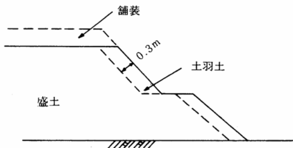
図 2-4-5 土羽土
