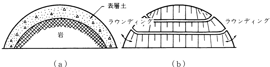
図2-3-4 縦断方向のラウンディング図
