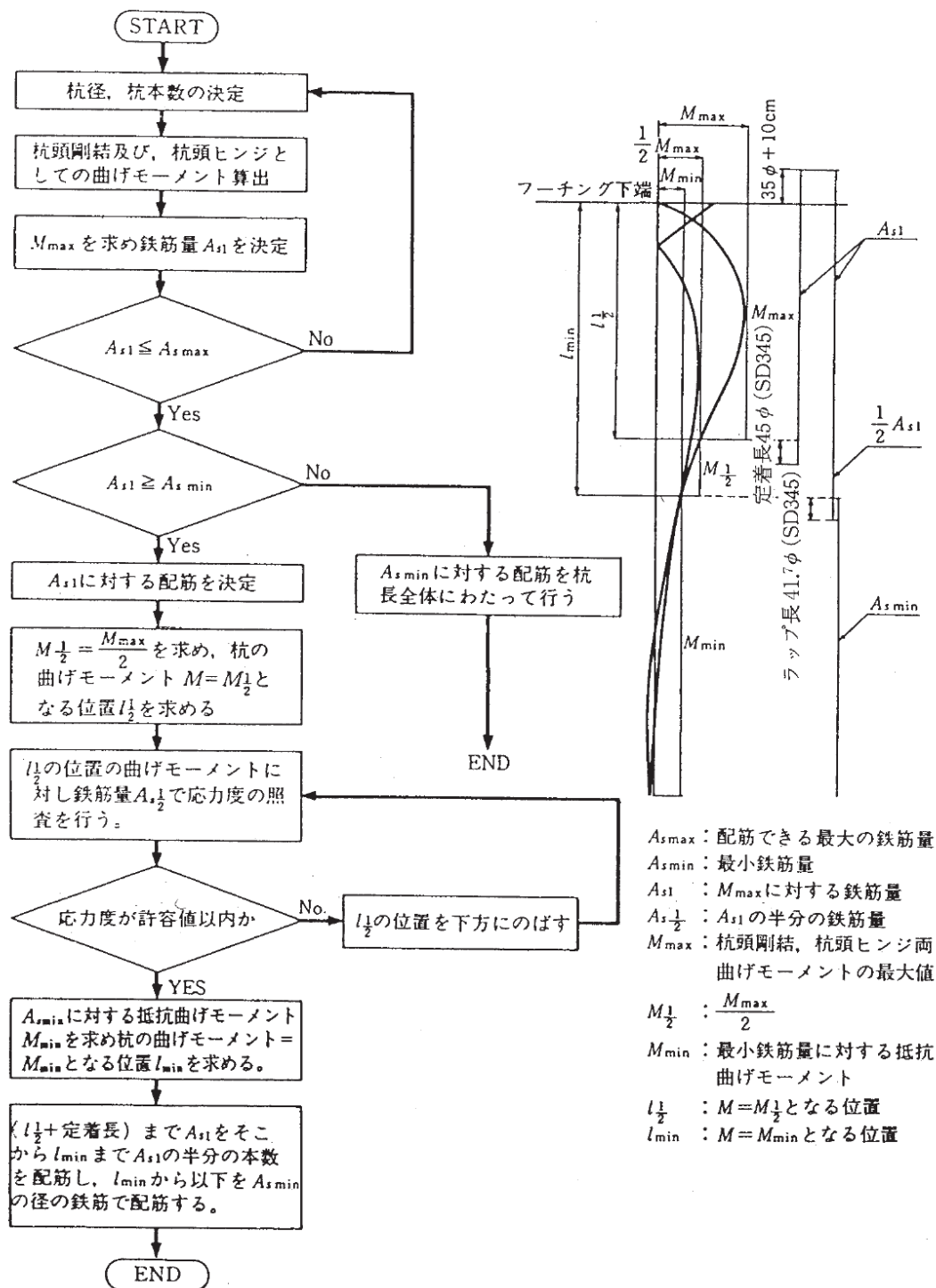
図4-1-14 主鉄筋断面変化図
