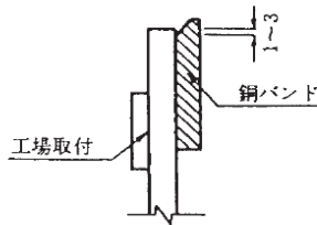
図 4-1-10 銅バンドの形状
