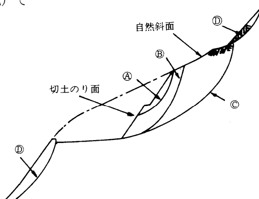
図2-3-7 掘削部の崩壊模式図
