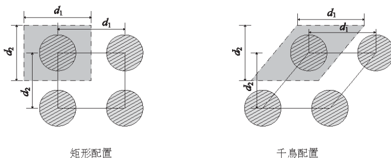
図3-2-6 改良体の配置
