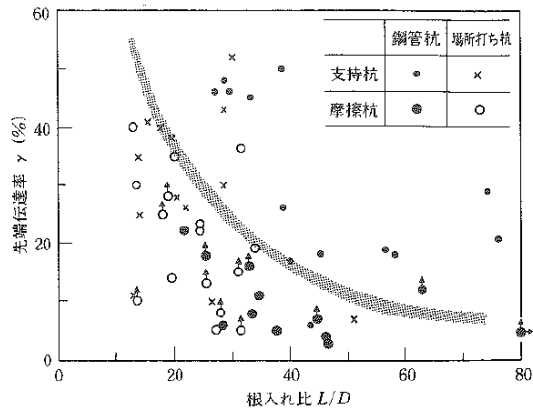
図4-1-7 先端伝達率 2)
