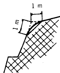
図2-3-3 のり肩のラウンディング標準図
