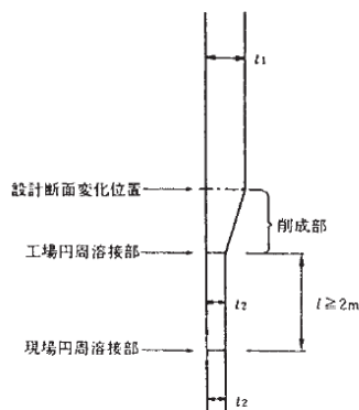
図 4-1-12 断面変化部の構造
