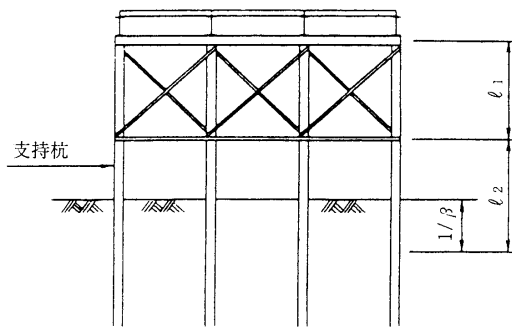
図 5-5-10 杭の座屈長
