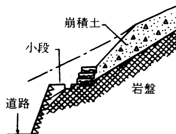
図2-3-6 崩壊対策図
