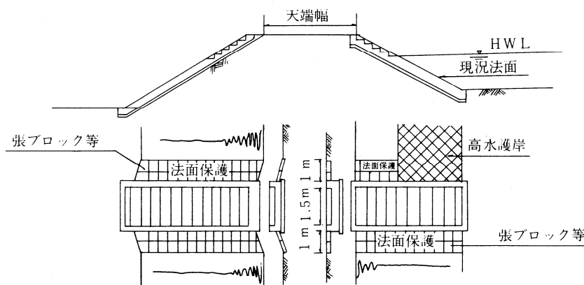
図 1-2-15 階段標準図
