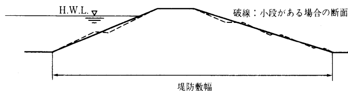
図 1-2-3 小段のあるのり面を緩勾配の一枚のりにする例
