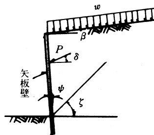
图 1-4-18 土压
