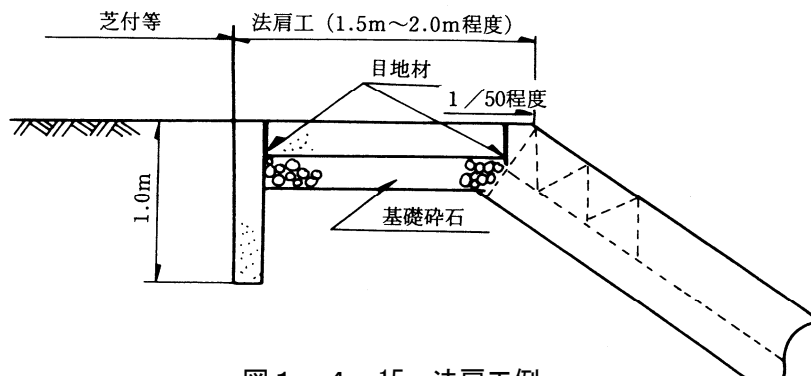
図1-4-15 法肩工例
