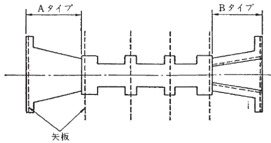
図 2-4-11 しゃ水矢板
