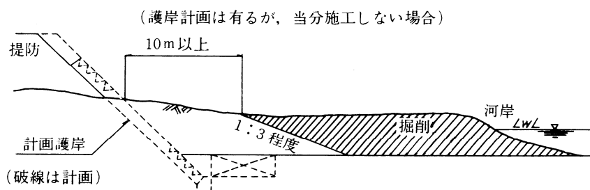
図 1-3-2 掘削(2)
