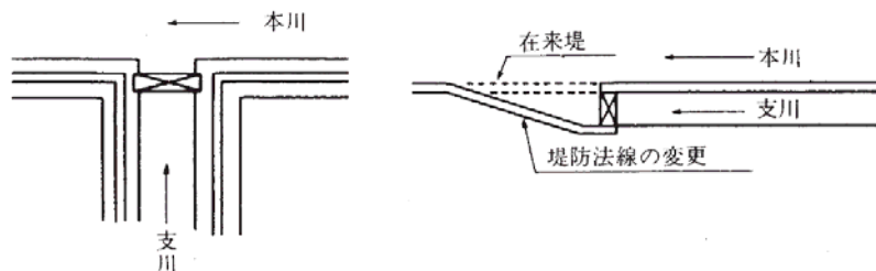
図3-1-1 水門設置位置
