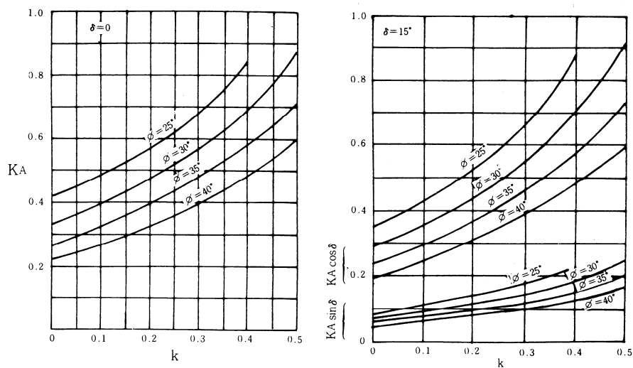
图 1-4-19 主动土压系数
