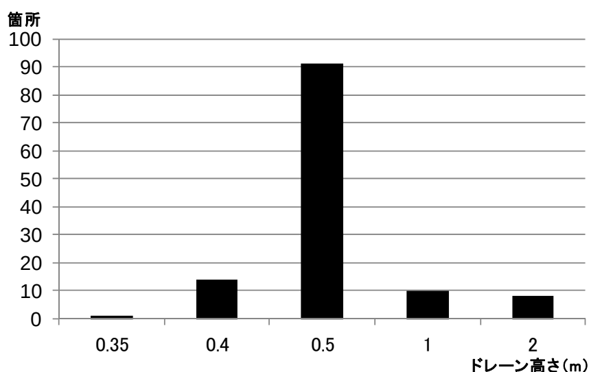
図 2.10 ドレーン工の高さ(厚み)の現地事例
