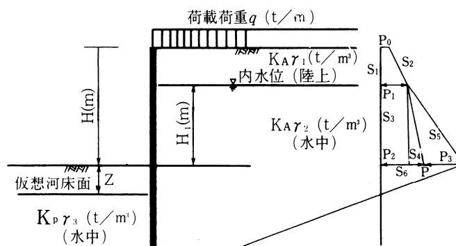
図 1-4-27 土圧、水圧
