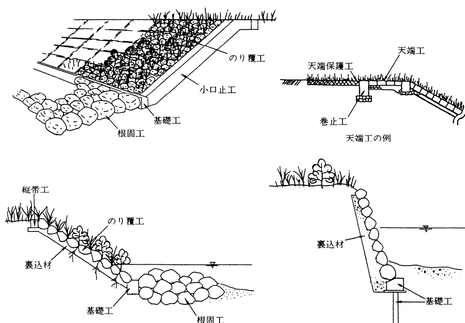
図 1-4-2 護岸の構成
