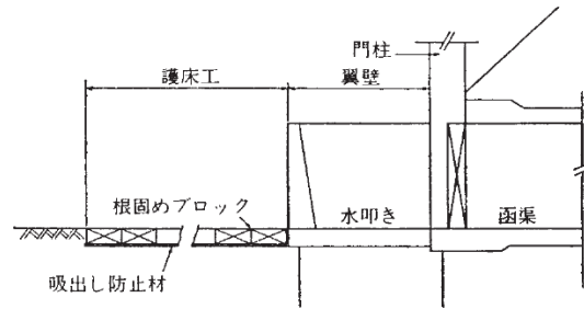
図 2-4-18 護床工（根固めブロックの例）
