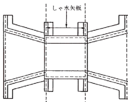
図3-2-2 水門のしゃ水矢板の配置
