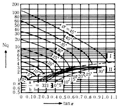
図 5-3-15 支持力係数 N_q を求めるグラフ
