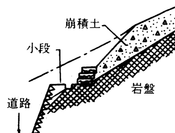
図 2-3-6 崩壊対策図
