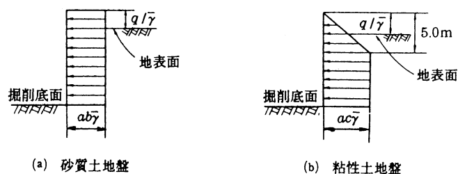
図 5-1-8 地表面での上載荷重がある場合の土圧
