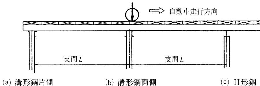
図 5-5-3 覆工受けたの支間長
