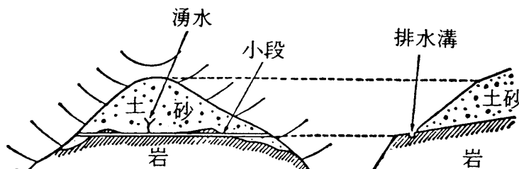
図2-3-2 小段の位置
