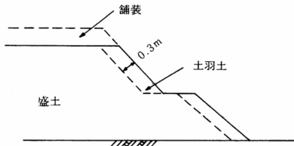
図2-4-5 土羽土
