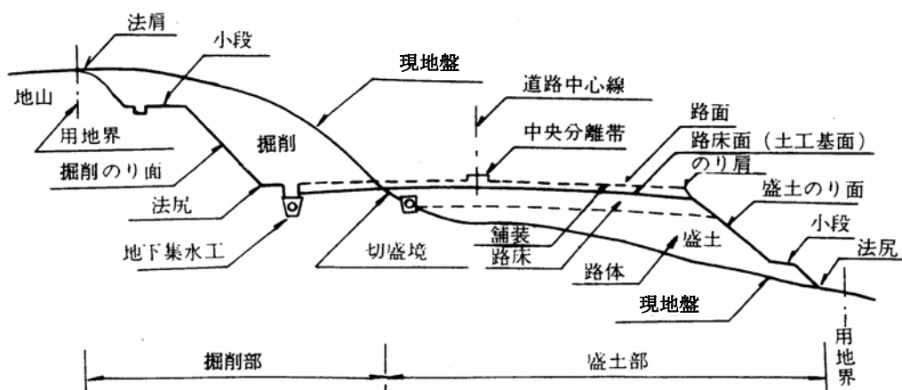
図 2-2-1 各部の名称
