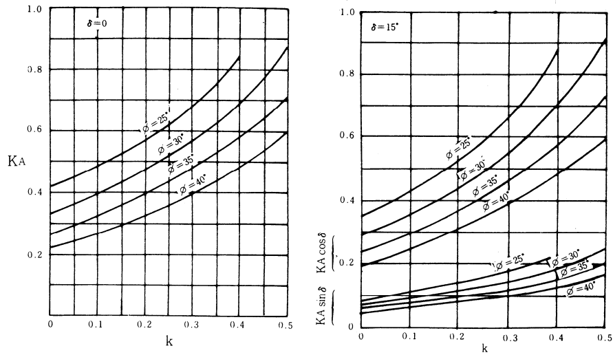
図 1-4-19 主動土圧係数
