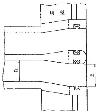
図2-4-4 二連以上の函渠端部
