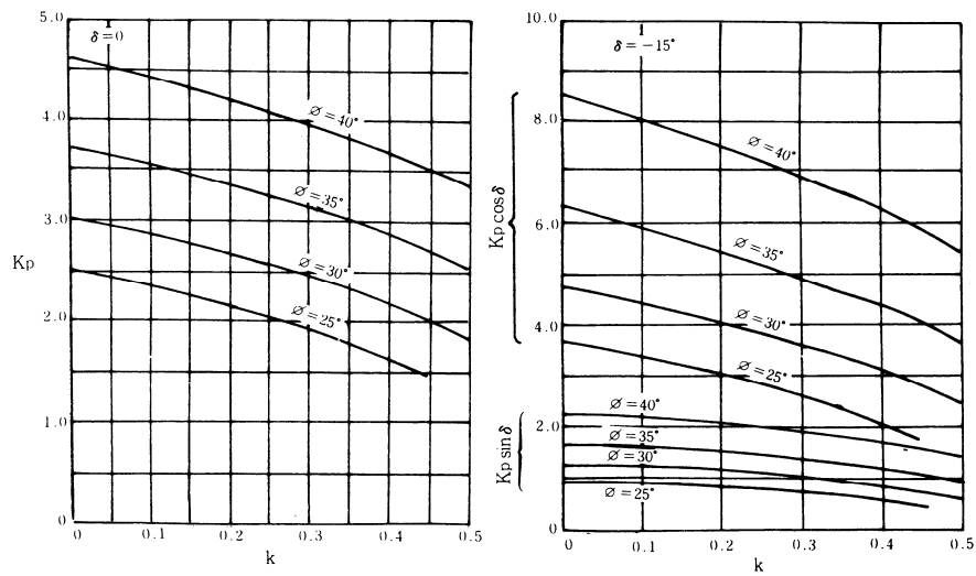
図 1-4-20 受働土圧係数
