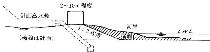
図1-3-1 掘削(1)
