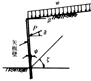
図 1-4-18 土圧
