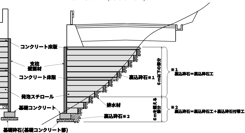
〔参考図 2 (片側壁面)〕
