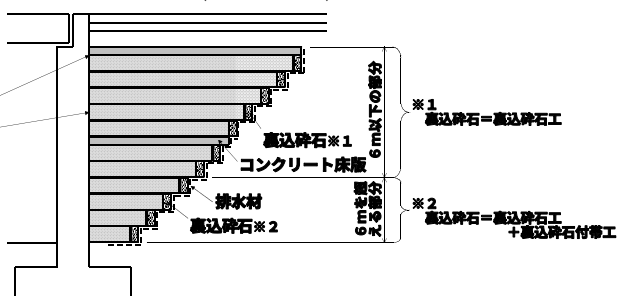
〔参考図 4 (橋台裏込)〕
