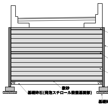
〔参考図 1 (両側壁面)〕
