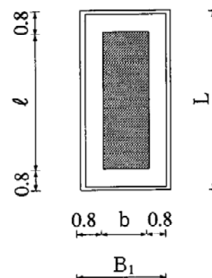
( 平 面 図 )
