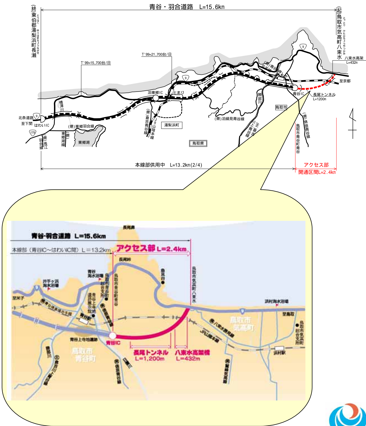
図-1 青谷・羽合道路全体図
