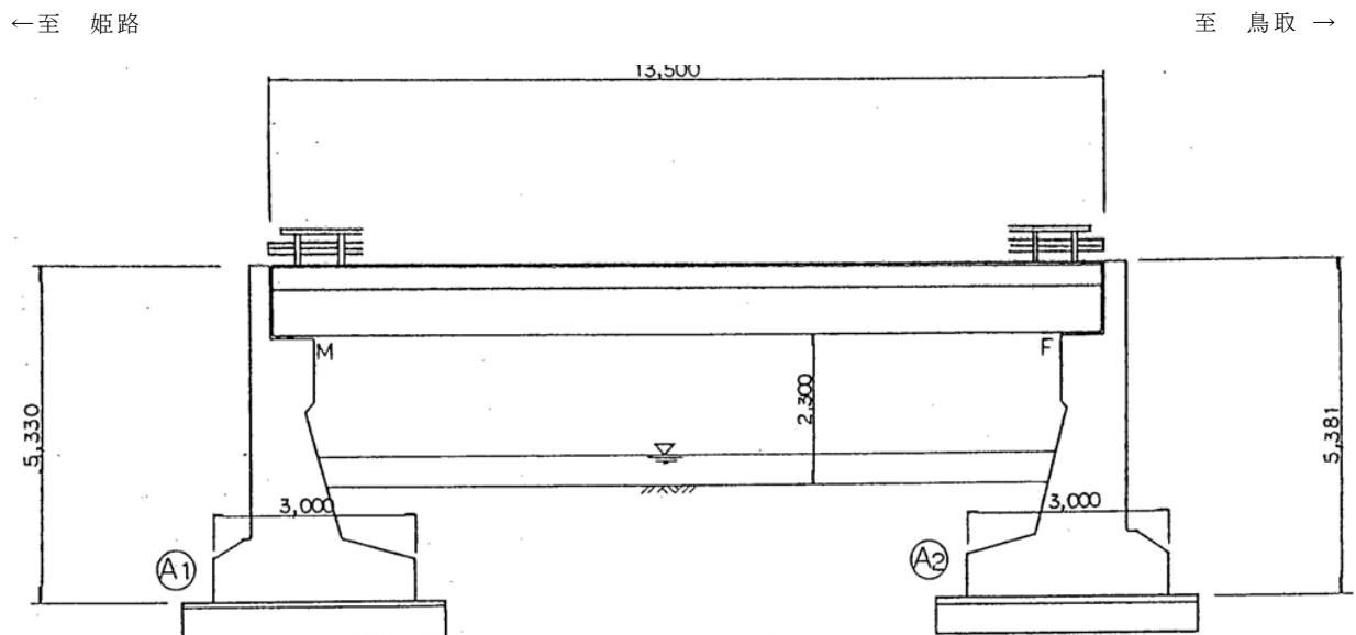
【橋梁側面図】
