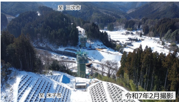
【写真①】 新屋地区の施工状況
