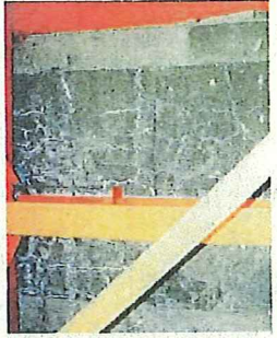
橋の裏面の様子(床版)
