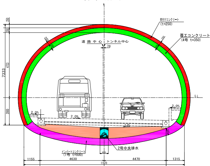
標準断面図
