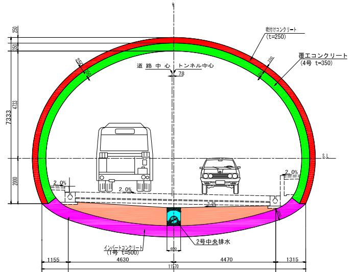
標準断面図
