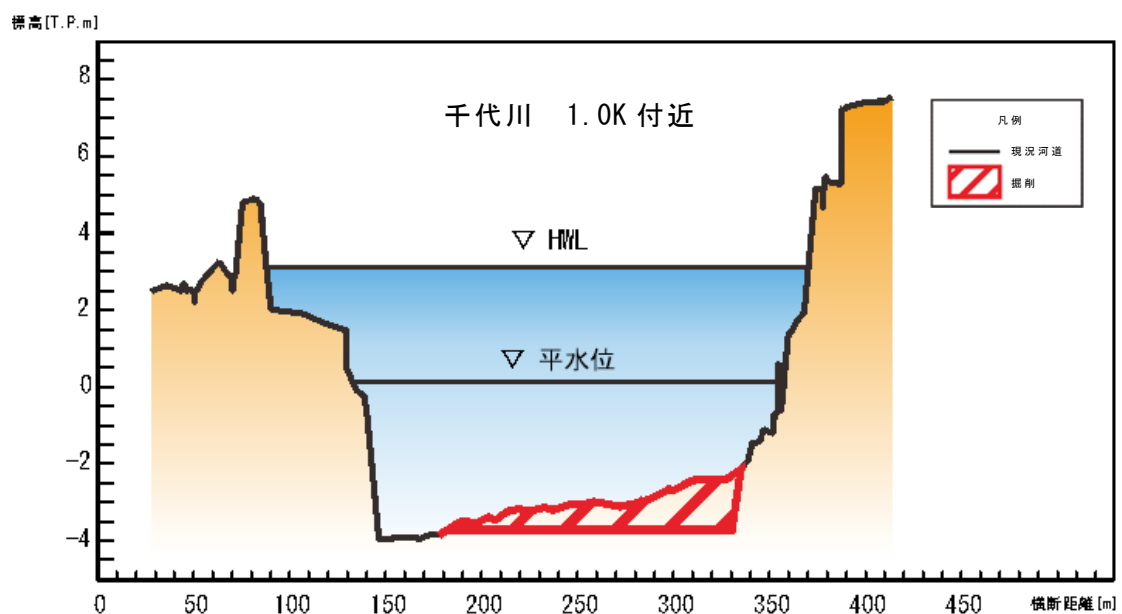
図 5.1.8 掘削のイメージ図
