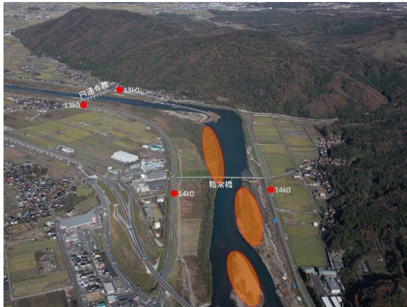
図 5.1.13 千代川 高水敷掘削・中州掘削の位置図 (13.5k~14.5k)
