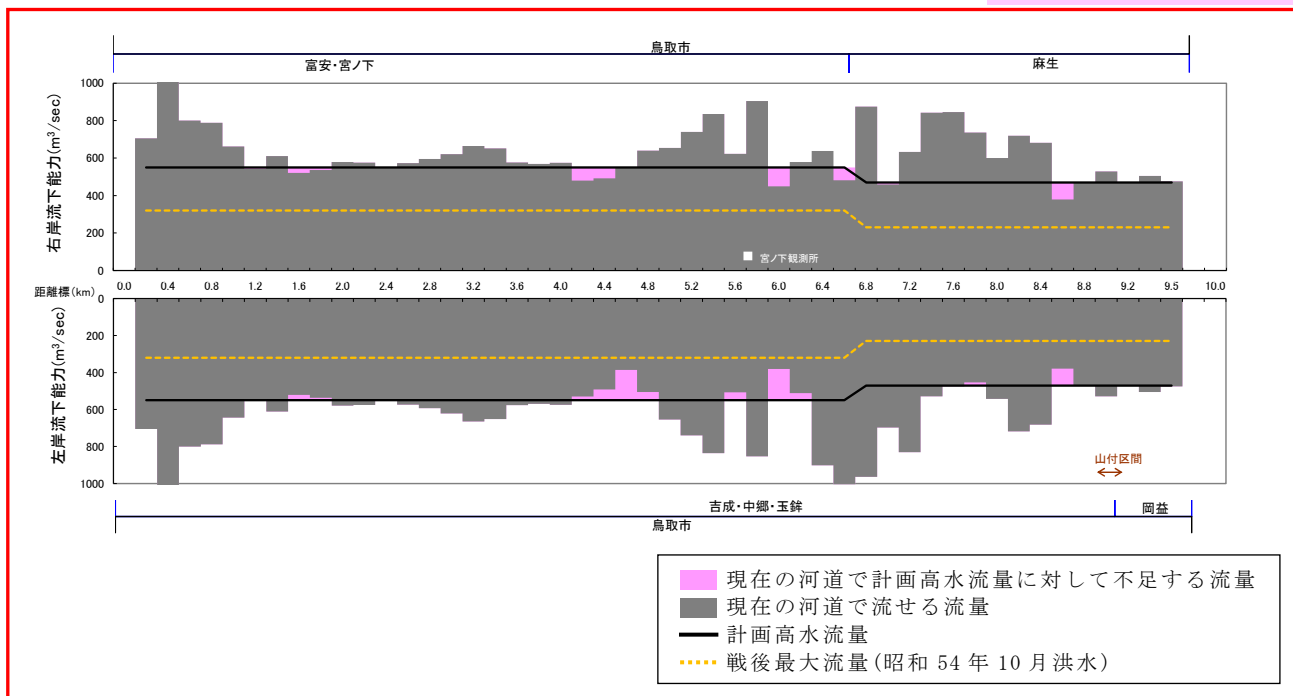
図 2.1.6 現在新袋川・袋川が安全に流すことの出来る流量
