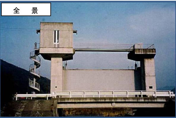
写真 2.4.5 樋門ゲートの劣化
