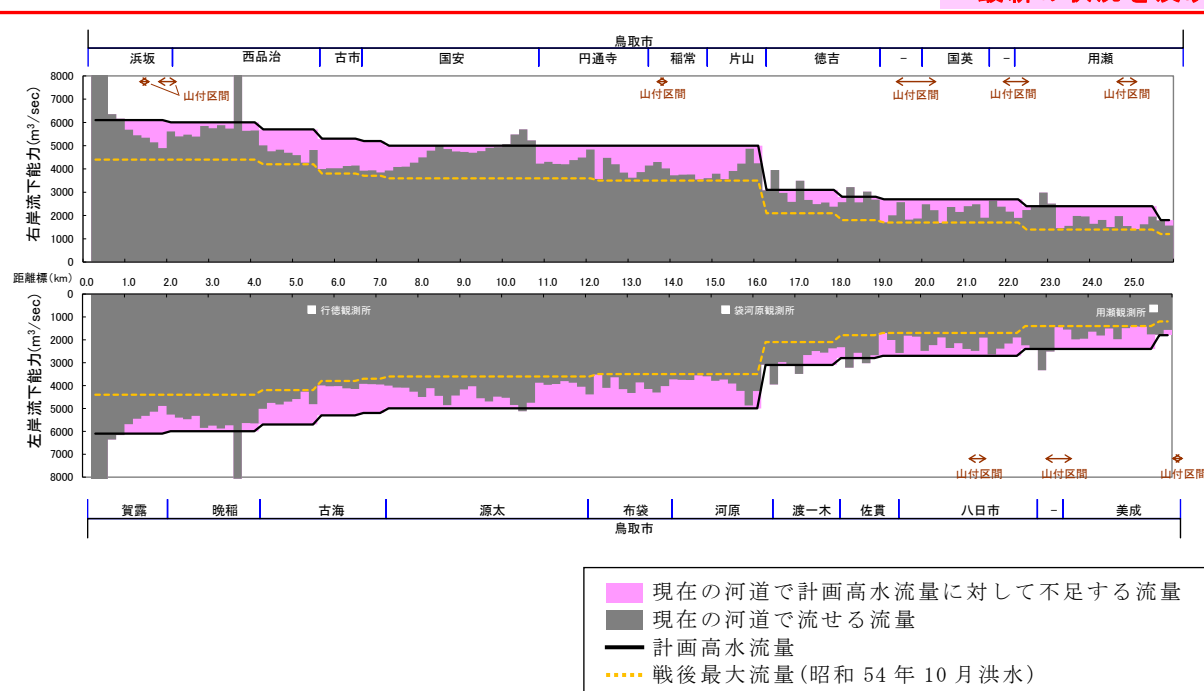
図 2.1.5 現在千代川が安全に流すことの出来る流量
