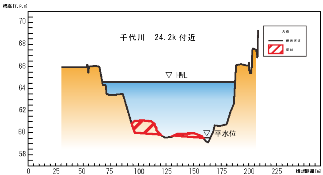
図 5. 1. 26 掘削のイメージ図
