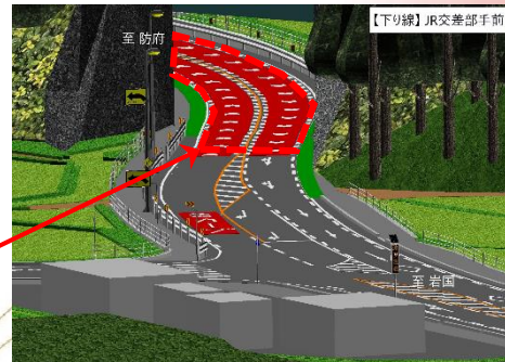
舗装改修箇所 (切削オーバーレイ・カラー舗装・区画線)
